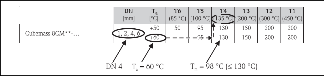
3: Procédure de détermination de la température de surface max.
