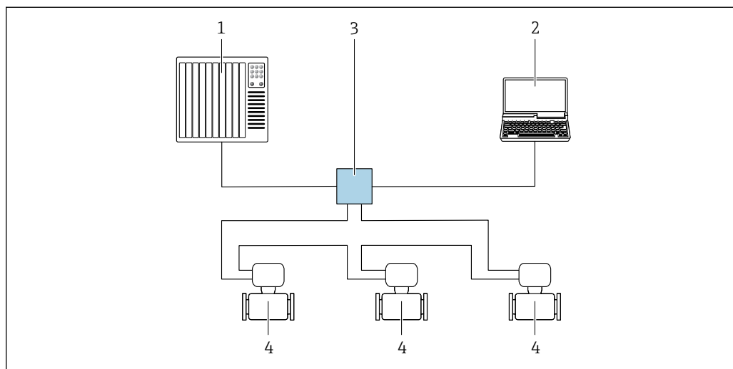
24 Варианты дистанционного управления через сеть PROFINET: топология «кольцо»
