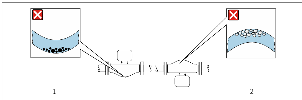
5 Монтажное положение датчика с изогнутой измерительной трубкой
