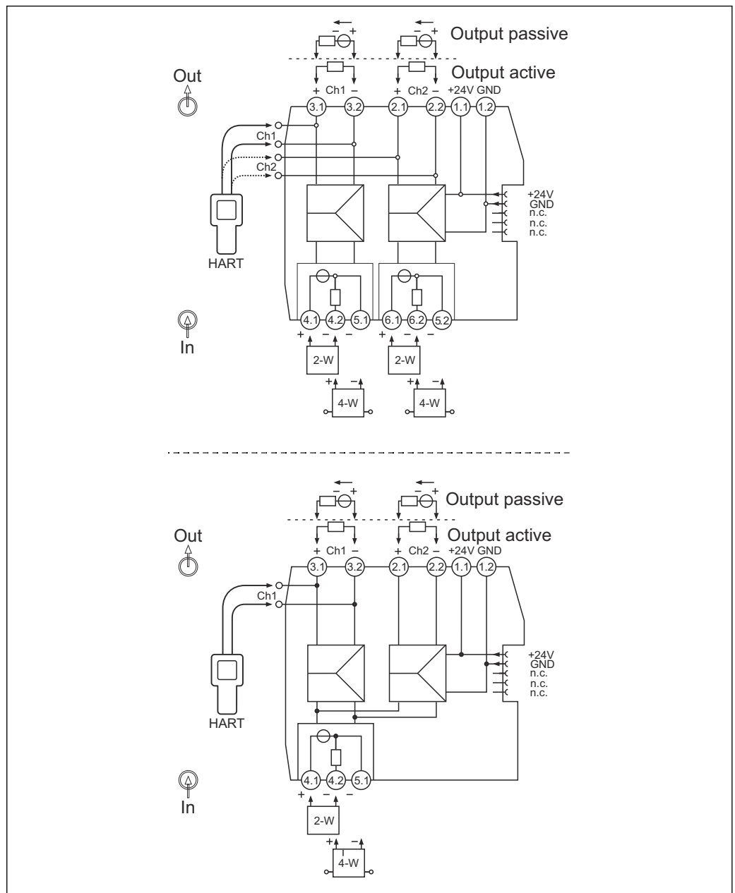
1 Klemmenbelegung: 1- und 2-Kanal Version (oben), Signaldoppler (unten)
