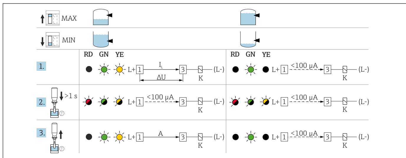
图 37 FEL62 的继电器响应和故障报警信号
