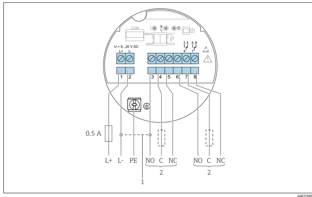
24 电子插件 FEL64 DC: 直流连接型, 带继电器输出
