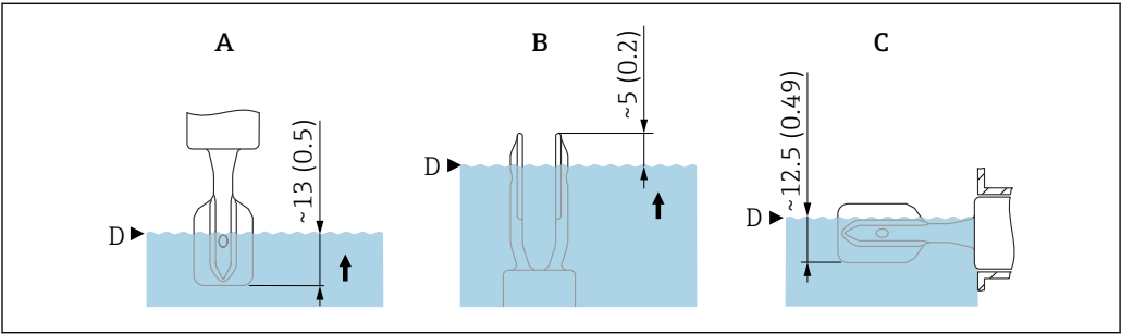
图 5 常见开关点。测量单位 mm (in)
