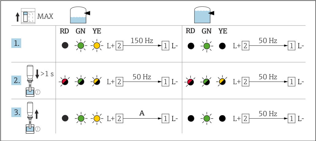
图 39 FEL67 在高限 (MAX) 检测模式下的继电器响应和故障报警信号
