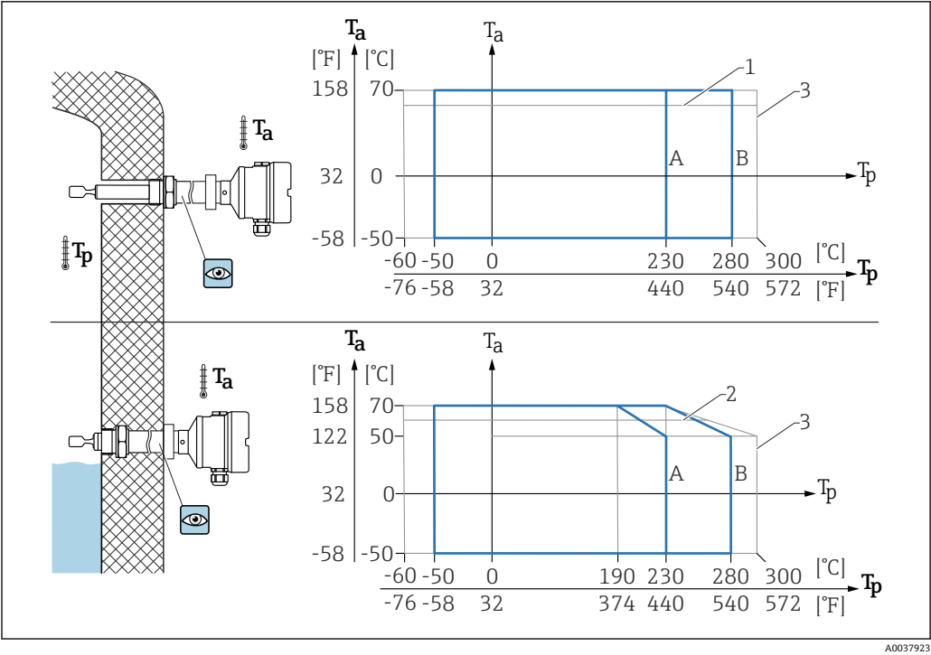
图 51 外壳允许环境温度 T_a 与罐体内部过程温度 T_p 的关系
