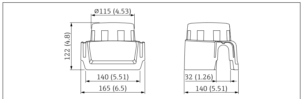
图 46 塑料防护罩 XW111 的外形尺寸示意图。测量单位 mm (in)
