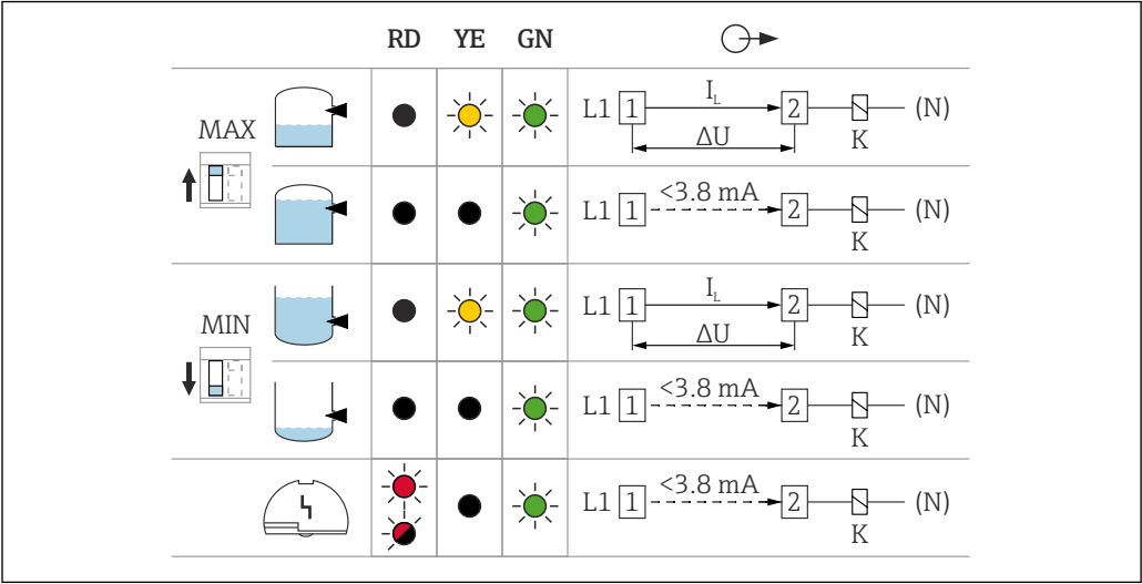
图 18 电子插件 FEL61 的继电器响应和故障信号
