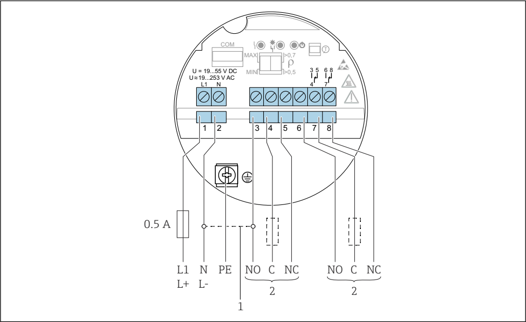
图 22 电子插件 FEL64：通用电流连接型，带继电器输出
