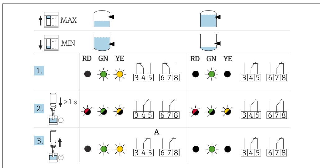
38 FEL64、FEL64DC 的继电器响应和故障报警信号
