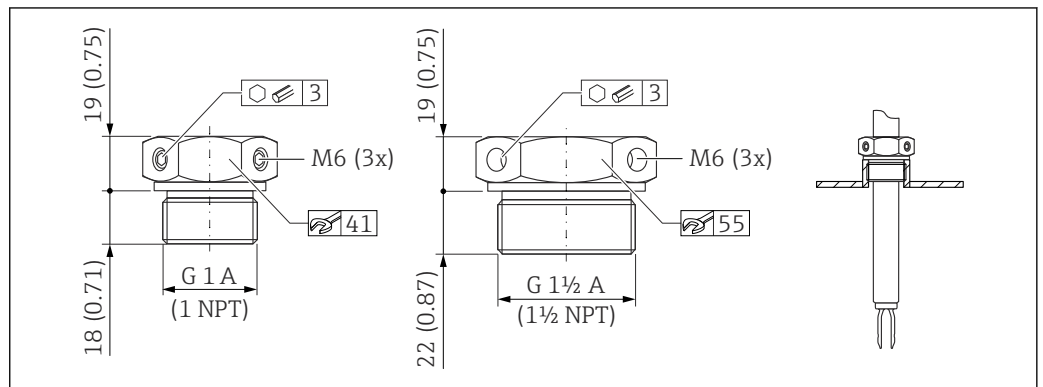
图 49 常压活动套管 p_e = 0 \text{ bar (0 psi)} 。测量单位 mm (in)
