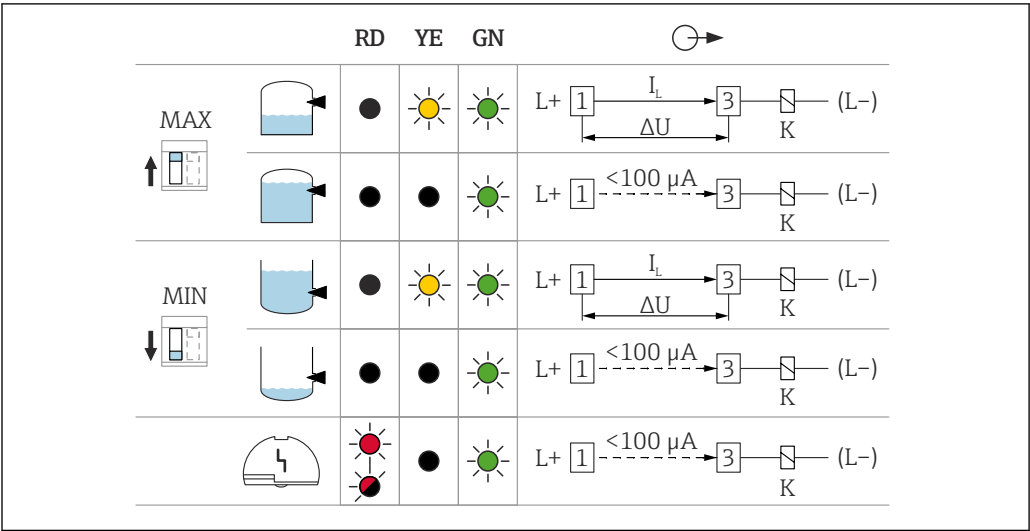
图 21 电子插件 FEL62 的继电器响应和故障信号
