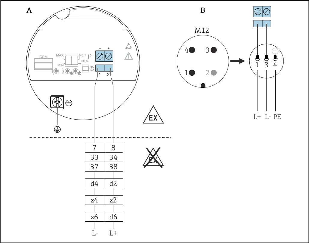
图 26 电子插件 FEL67: PFM 输出
