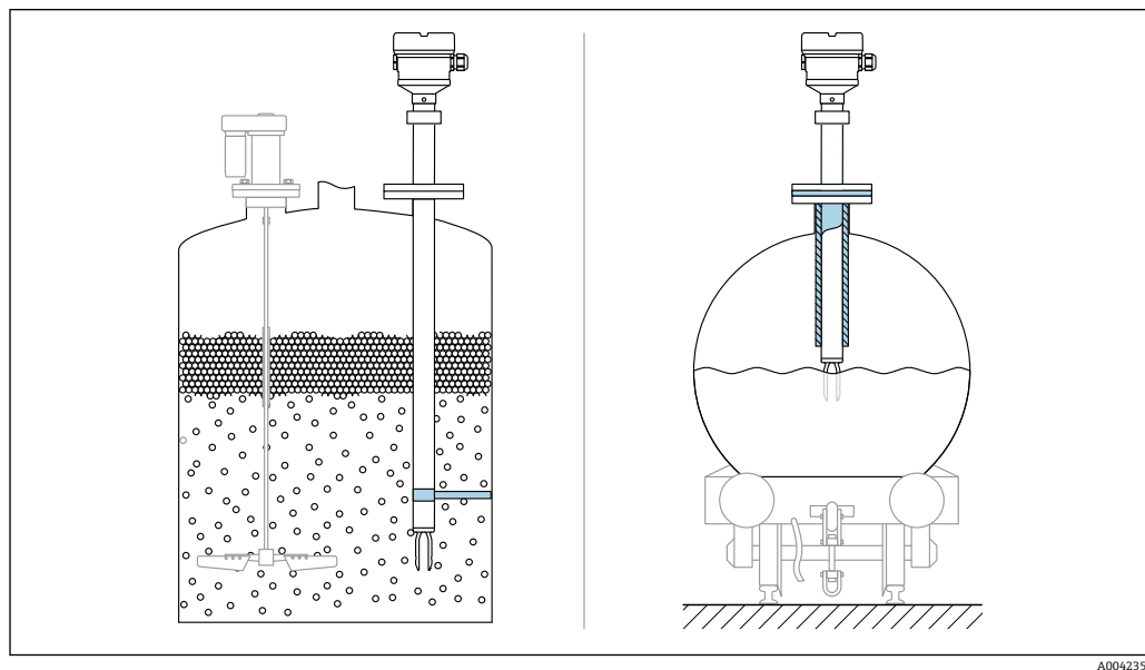
图 10 实例：存在动态负载时，应支撑设备
