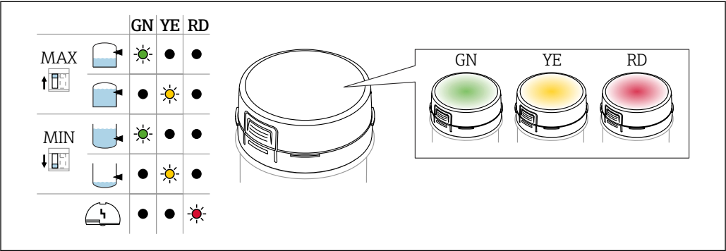
图 30 LED 指示灯以绿色 (GN)、黄色 (YE) 或红色 (RD) 醒目显示
