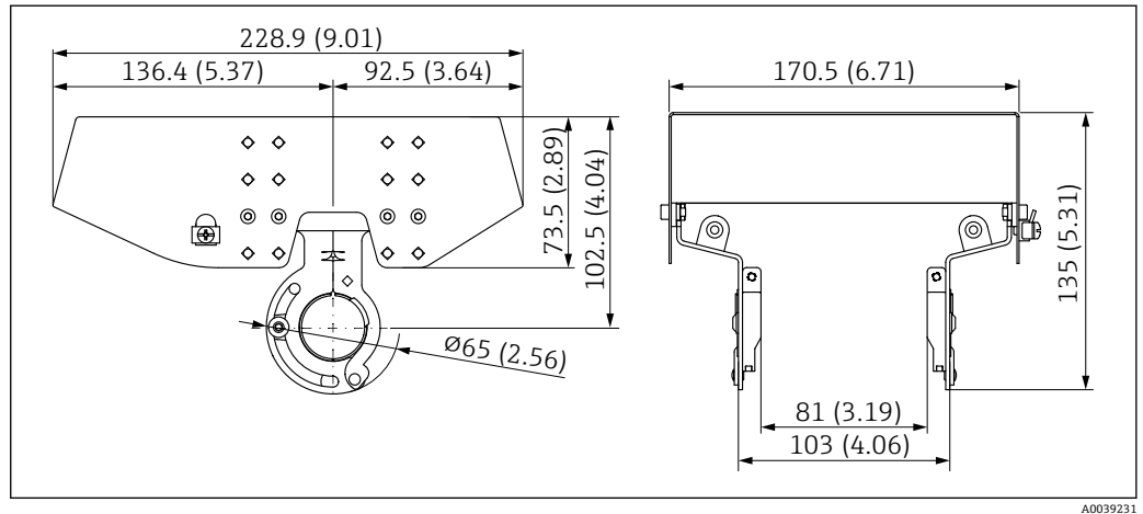
图 45 316L 防护罩 XW112 的外形尺寸示意图。测量单位 mm (in)
