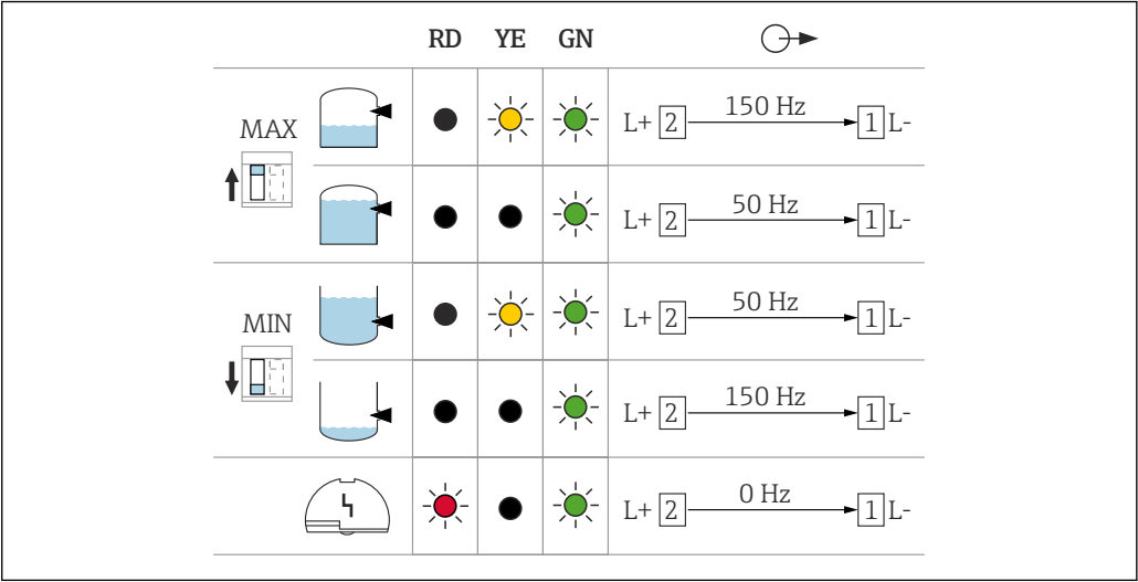
图 27 电子插件 FEL67 的继电器响应和故障信号
