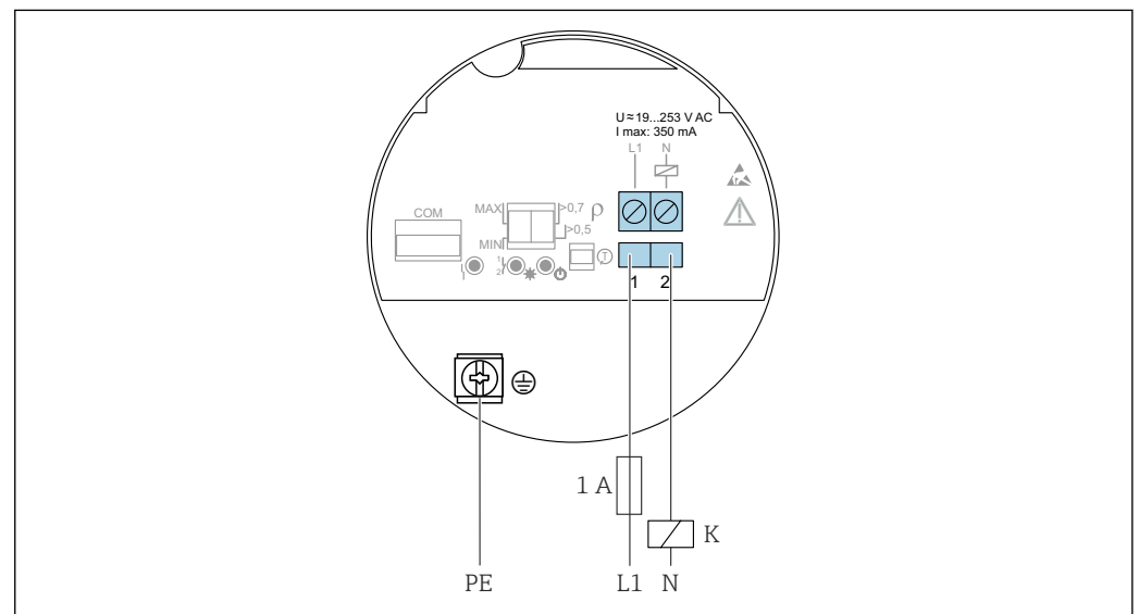
17 FEL61 电子插件: 两线制连接, 交流 AC 型
