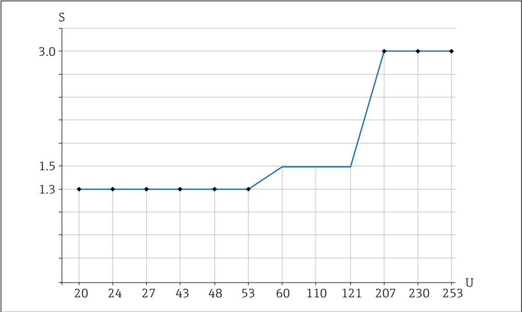
图 19 负载的推荐最小持续功率/额定功率
