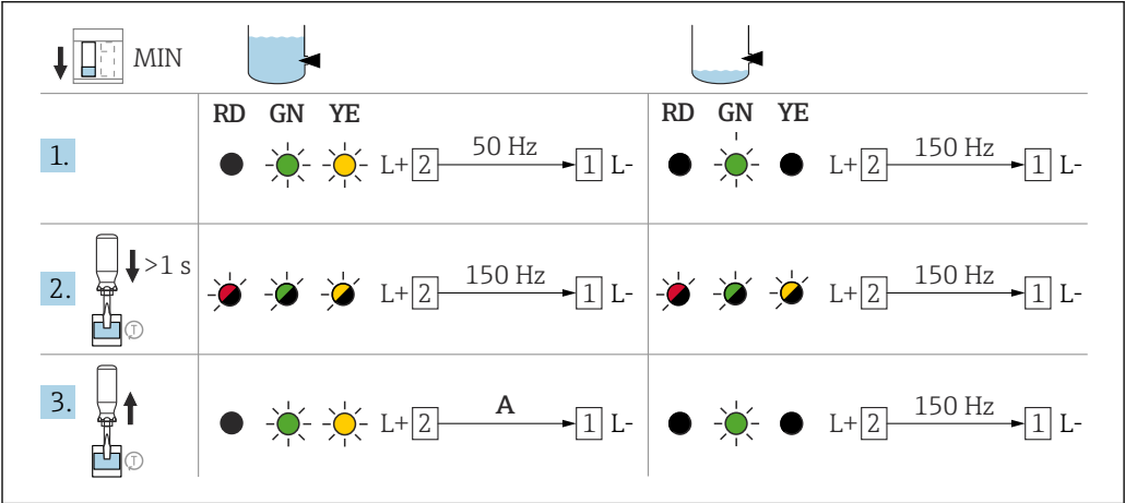
图 40 FEL67 在低限 (MIN) 检测模式下的继电器响应和故障报警信号
