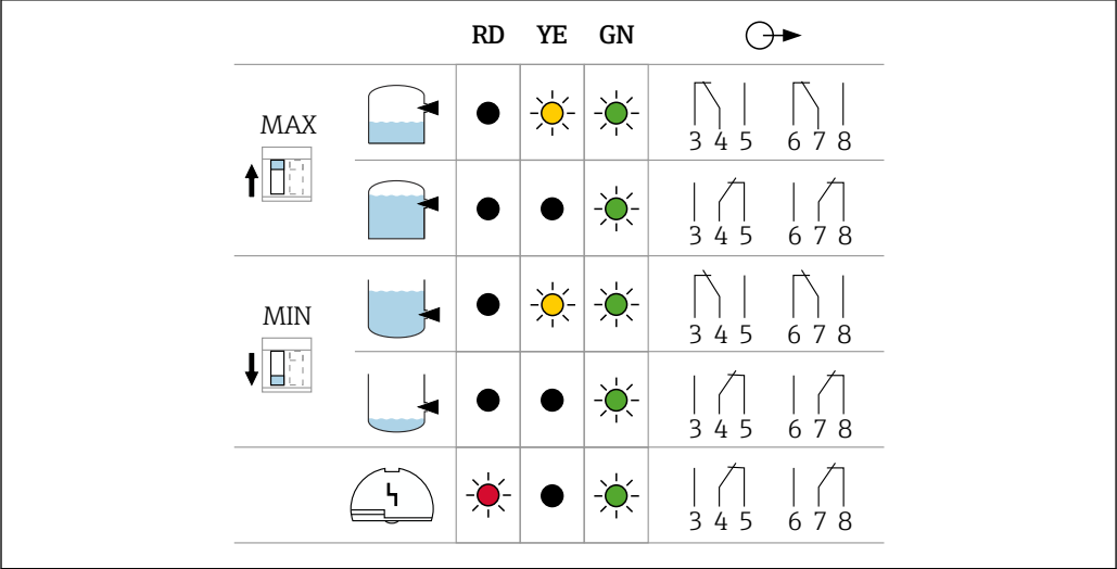
图 23 电子插件 FEL64 的继电器响应和故障信号
