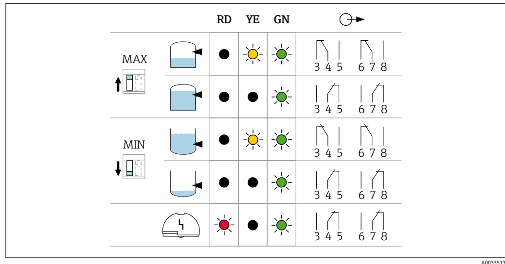
25 电子插件 FEL64 DC 的继电器响应和故障信号
