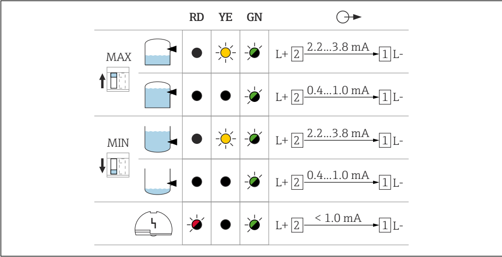
图 29 电子插件 FEL68 的开关量输出和信号传输
