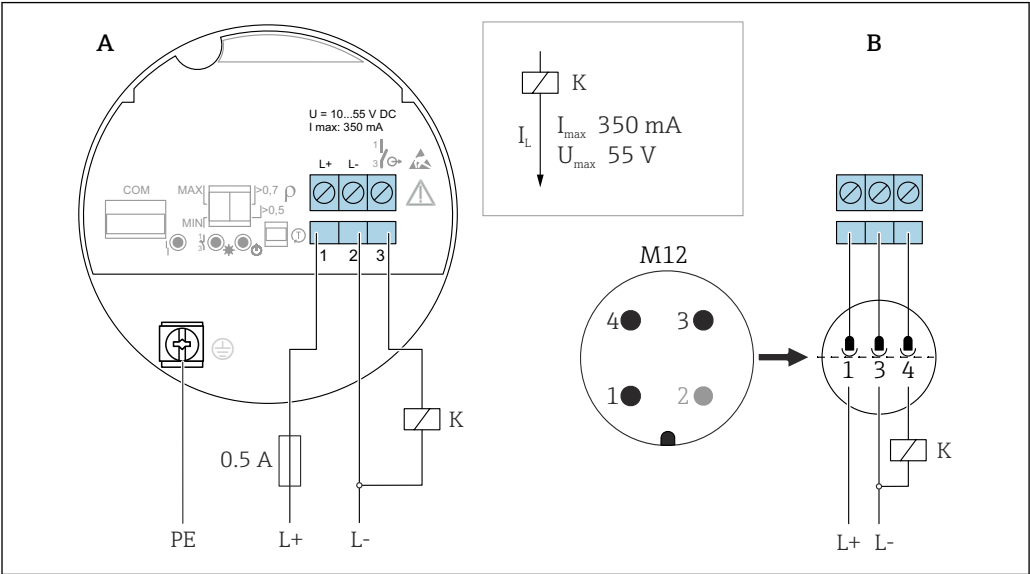
图 20 电子插件 FEL62: 三线制连接, 直流 DC-PNP 型
