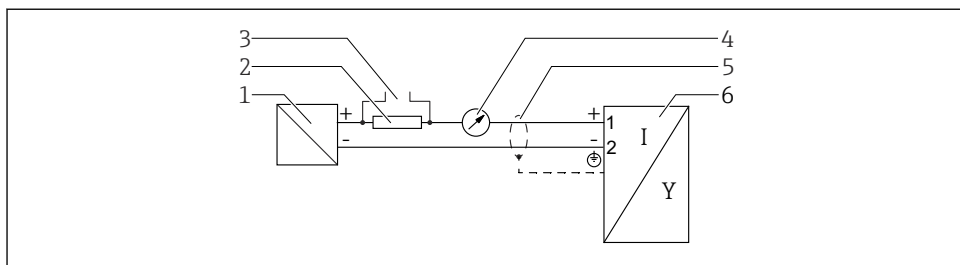
6 Diagrama de função HART 4 para 20 mA
