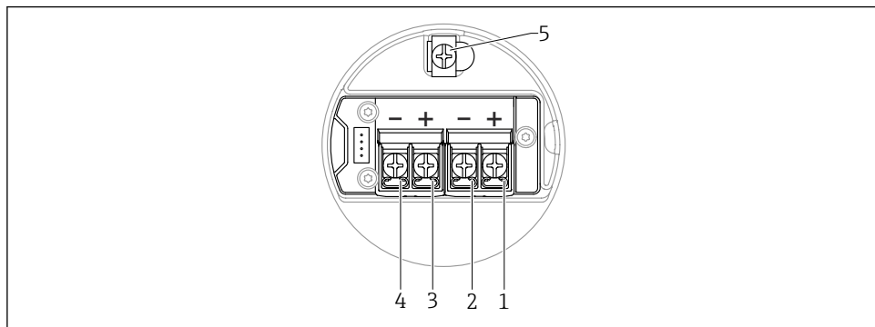
16 Esquema de ligação elétrica no compartimento de conexão; HART 4 para 20 mA + analógica 4 para 20 mA; invólucro de compartimento duplo em formato de L
