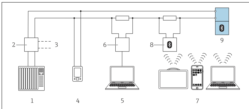
21 Opções para operação remota através do protocolo HART
