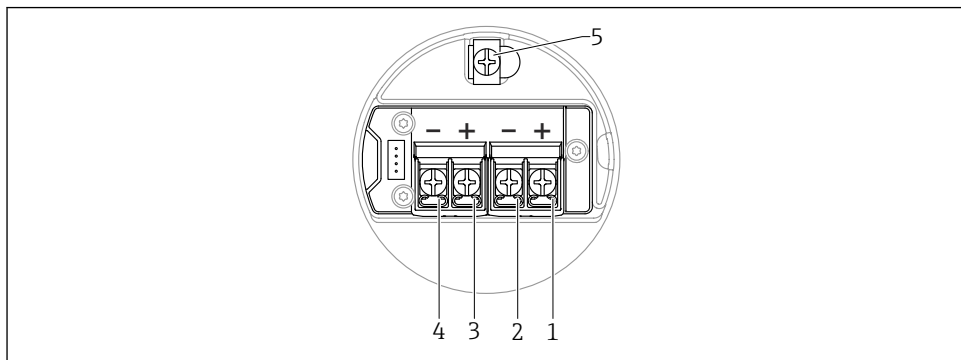
17 Esquema de ligação elétrica no compartimento de conexão; HART 4 para 20 mA, saída comutada, invólucro de compartimento duplo em formato de L
