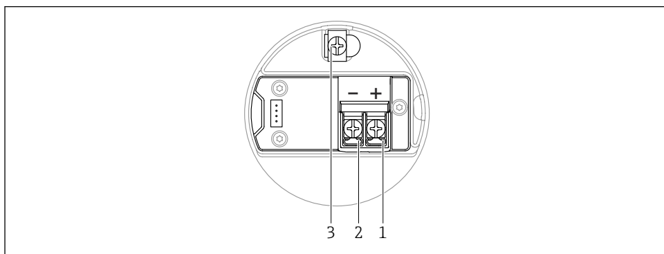
15 Esquema de ligação elétrica no compartimento de conexão; HART 4 para 20 mA, Invólucro de compartimento duplo em formato de L
