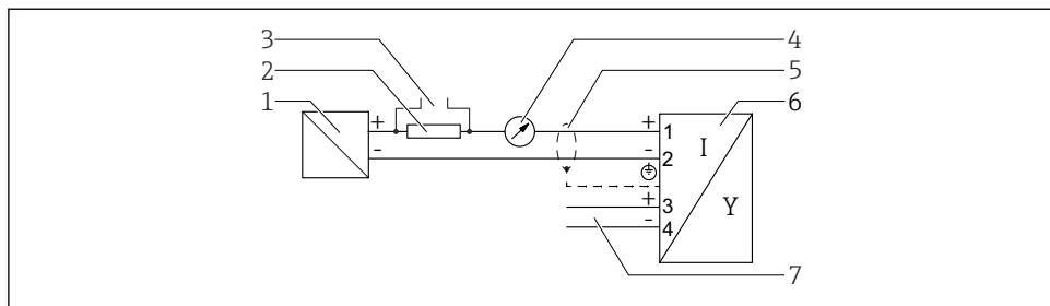
7 Diagrama de função HART 4 para 20 mA, saída comutada
