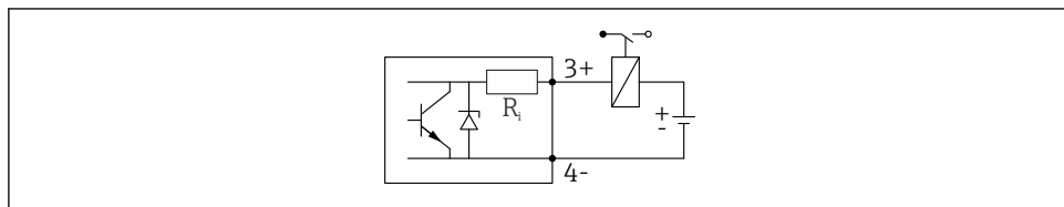
8 Exemplo de conexão de um relé
