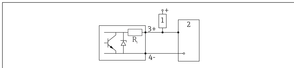
9 Exemplo de conexão para a entrada digital
