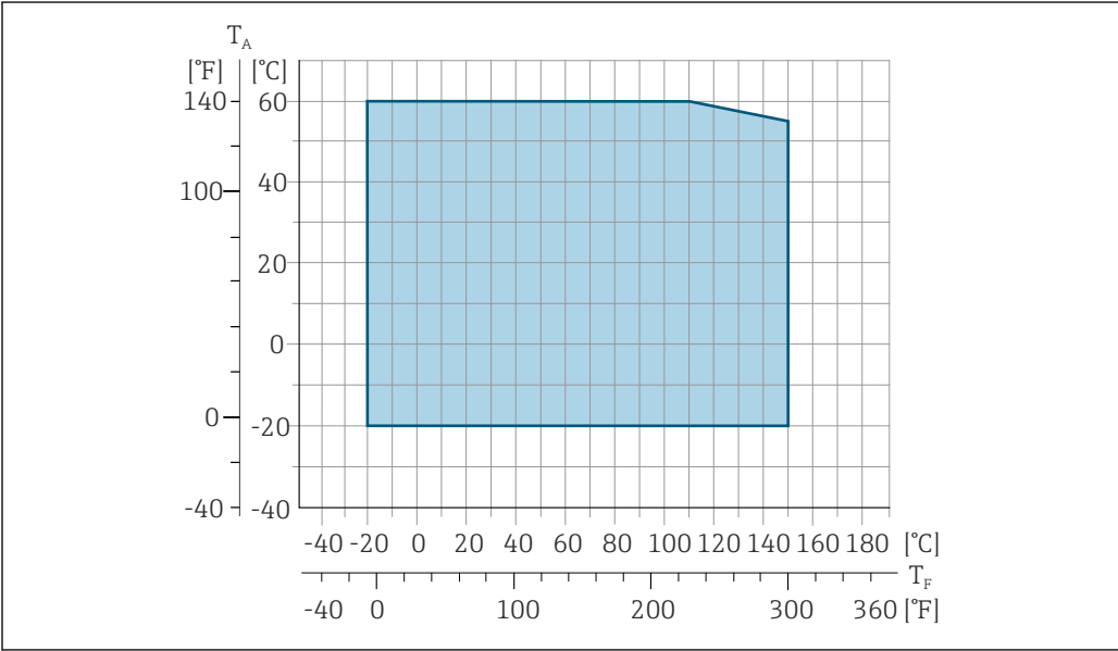
图 41 Promag 500 (模拟)
