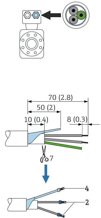
供电电缆
