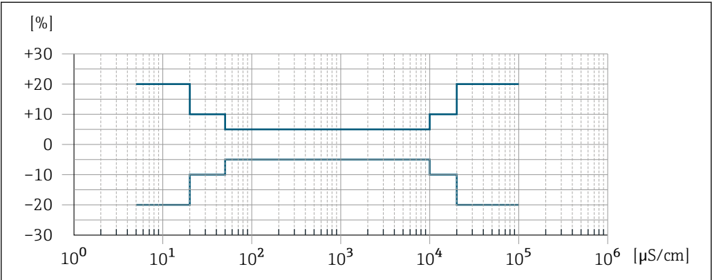
图 39 测量误差 (可选: 订购选项“电导率测量标定”，选型代号 CW)
