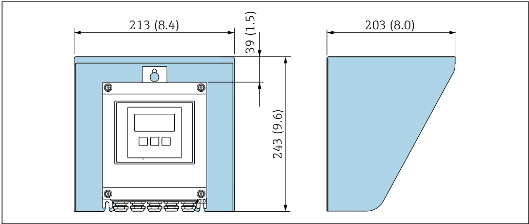
图 7 Proline 500（数字）变送器的防护罩；单位：mm (in)
