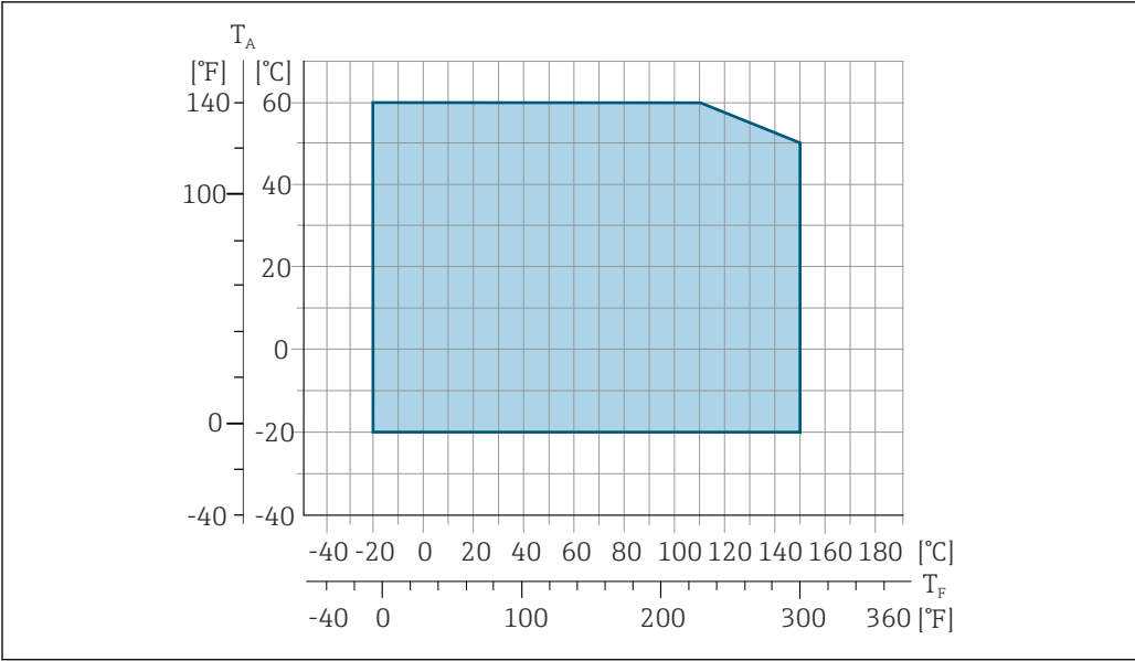
图 40 Promag 500 (数字)
