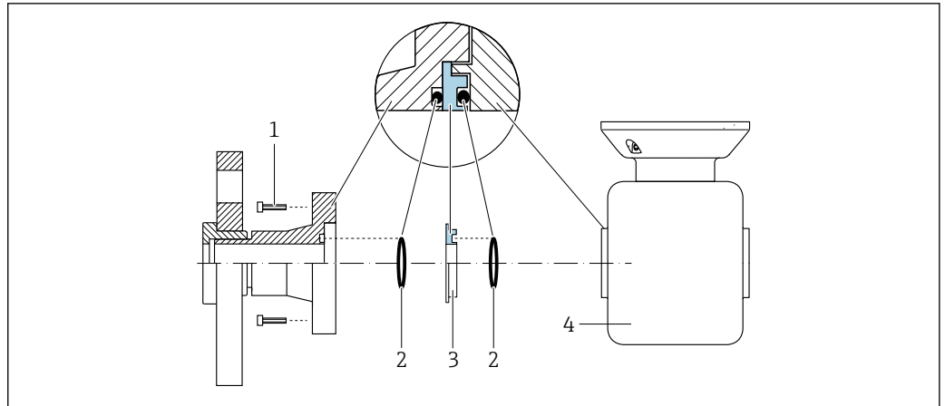
图 9 安装接地环
