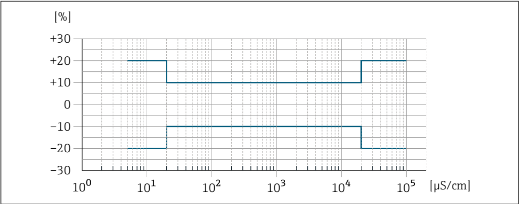
图 38 测量误差 (标准)
