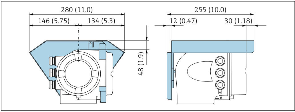
图 8 Proline 500 变送器的防护罩；单位：mm (in)
