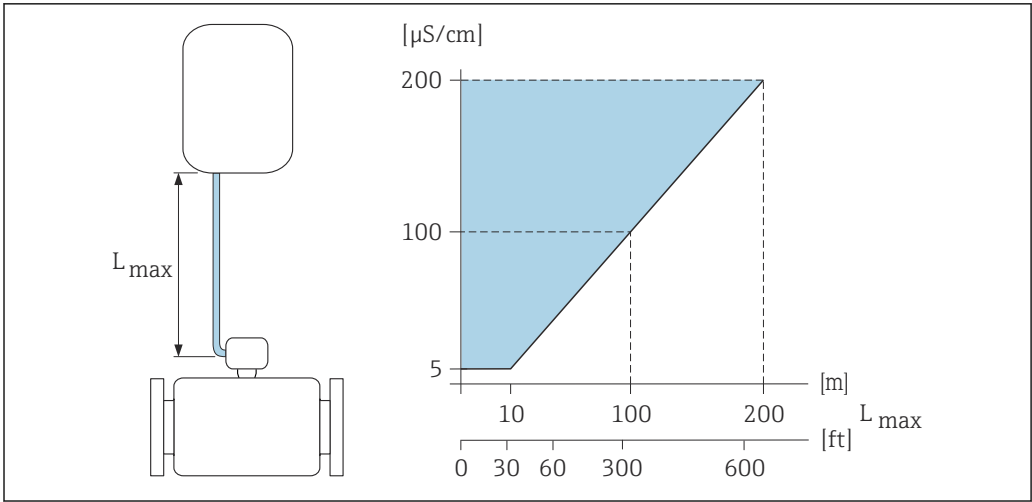
图 6 允许连接电缆长度 彩色区域 = 允许电缆长度范围 L_{\max} = 连接电缆长度 ([m] ([ft]) ) [ \mu S/cm] = 介质电导率
