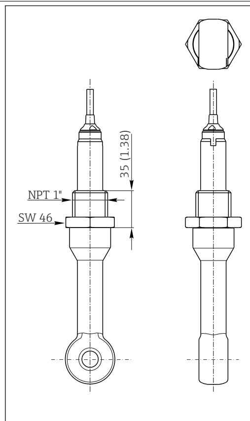
17 Version, filetage NPT 1". Unité de mesure mm (in)
