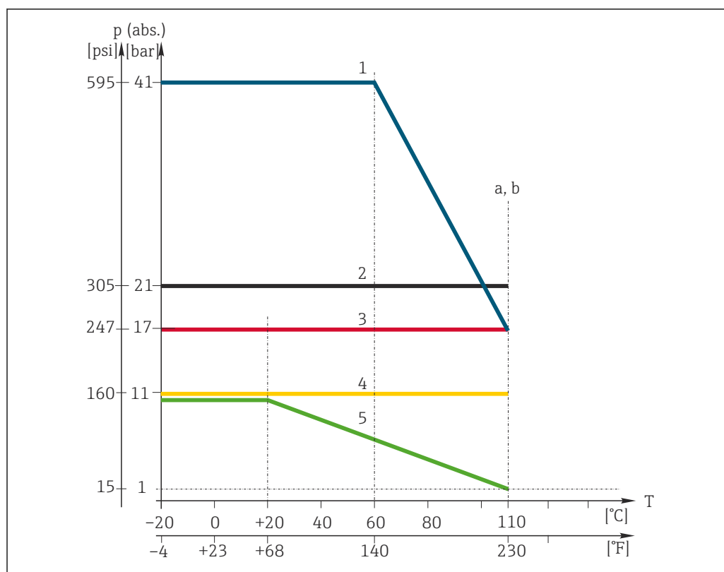
11 Courbes de température/pression
