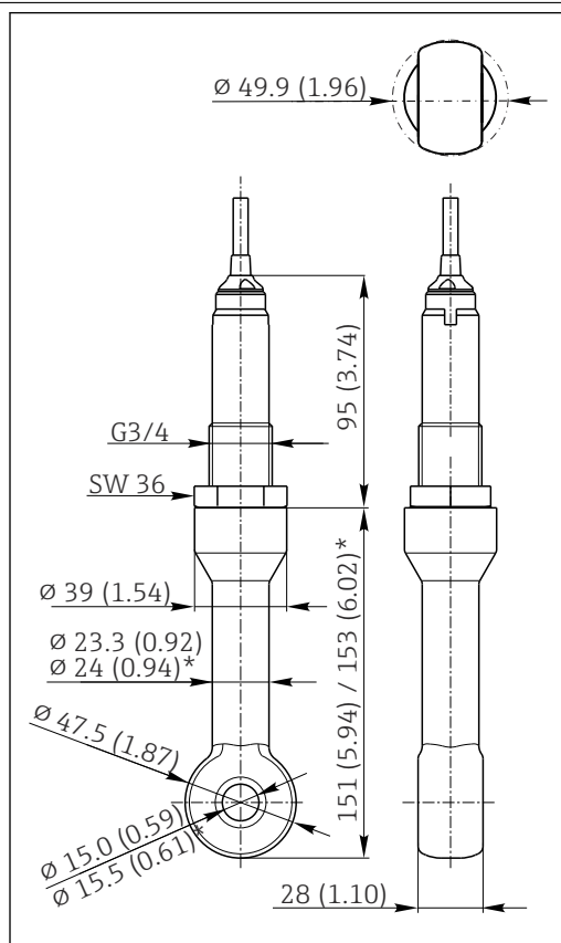
16 Version avec filetage G \frac{3}{4} . Unité de mesure mm (in)
