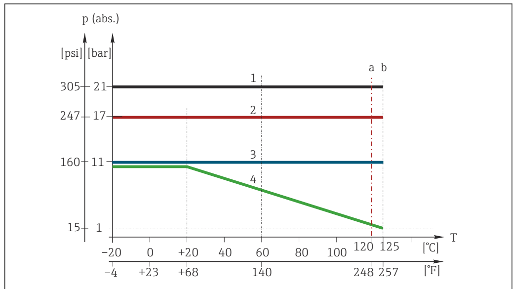
12 Courbes de température/pression
