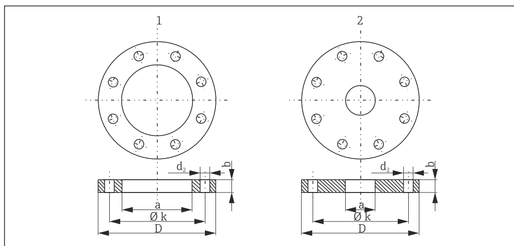
19 Dimensions des brides
