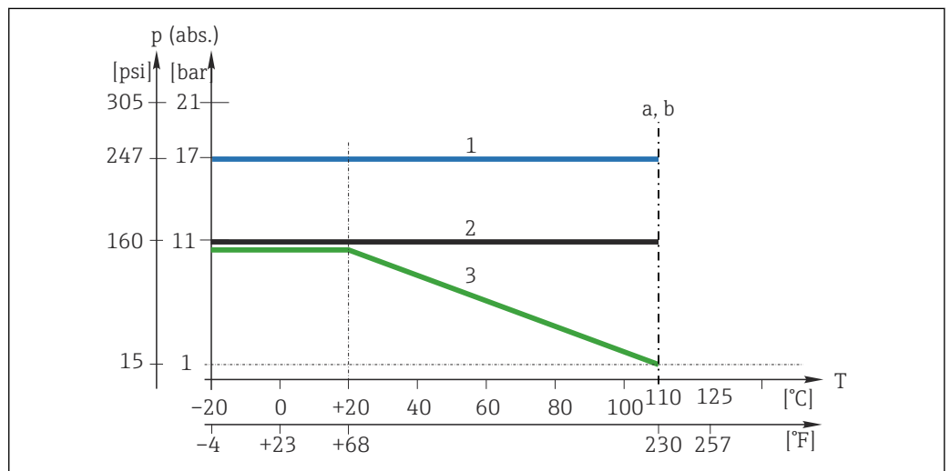
13 Courbes de température/pression
