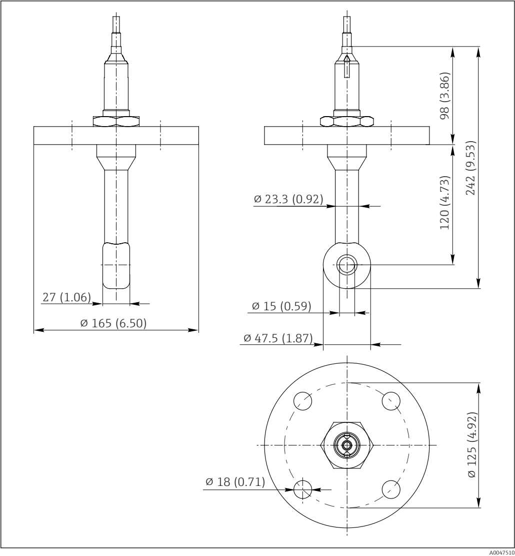
18 Version, bride EN1092-1 DN50 PN16, 316L, plaque d'étanchéité PFA du capteur soudée. Unité de mesure mm (in)
