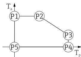
36 Invólucro plástico; temperatura do processo 0 para +200 °C (+32 para +392 °F) com aprovação CSA C/US
