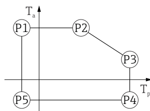
35 Invólucro plástico; temperatura do processo -40 para +200 °C (-40 para +392 °F)
