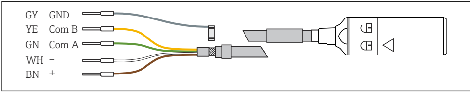
10 Кабель передачи данных Memosens CYK10
