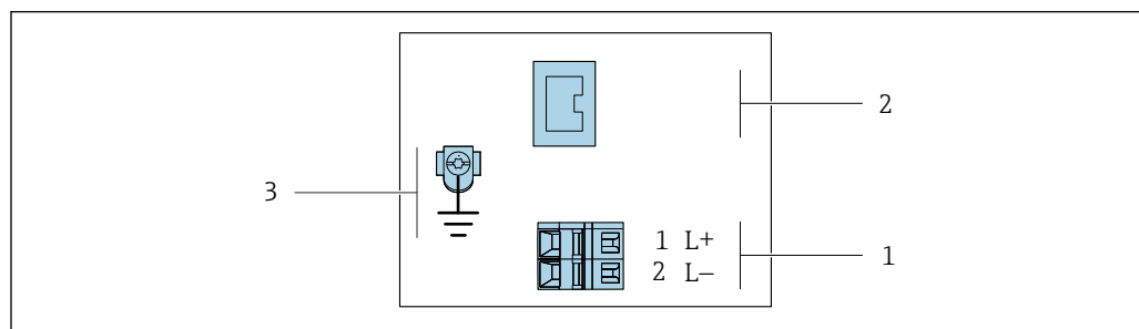
7 PROFINET 端子の割当て
