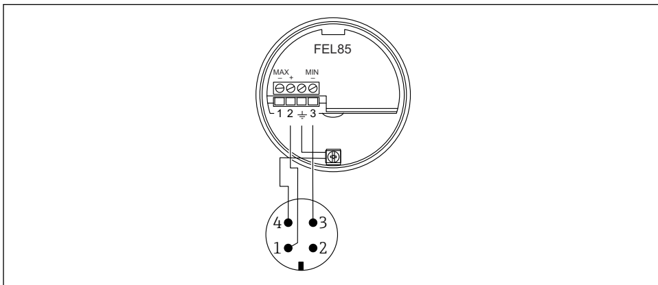
17 Schemat styków złącza M12, tryb sygnalizacji MIN
