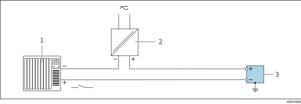
図 22 ステータス入力の接続例 1 オートメーションシステム、スイッチ出力（パッシブ）付き（例：PLC） 2 電源 3 ステータス入力付き変換器
