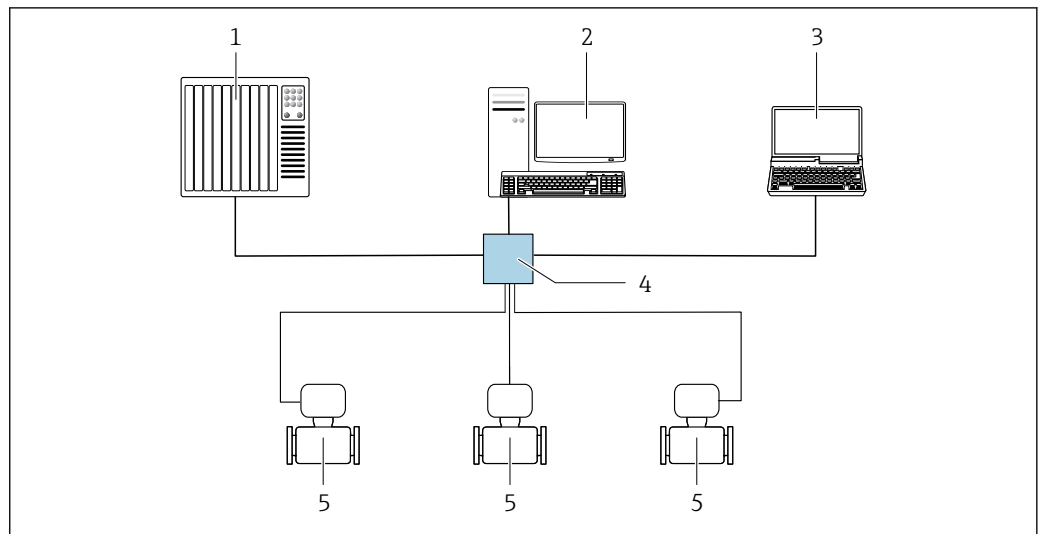
54 Opções para operação remota através do Modbus TCP por Ethernet - 100 Mbit/s: Topologia estrela
