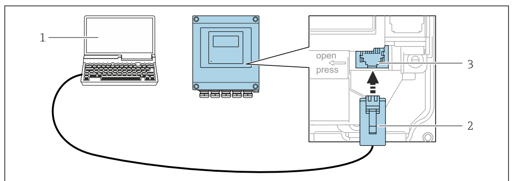
55 Conexão através de Interface de operação (CDI-RJ45)
