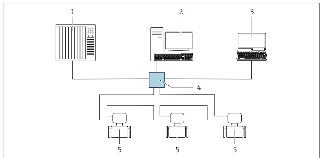
50 Opções para operação remota através da rede EtherNet/IP: topologia de anel
