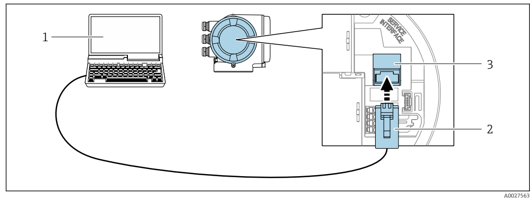
56 Conexão através de Interface de operação (CDI-RJ45)
