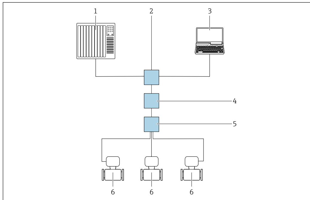
53 Opções para operação remota através do protocolo Modbus TCP por Ethernet-APL (ativa)
