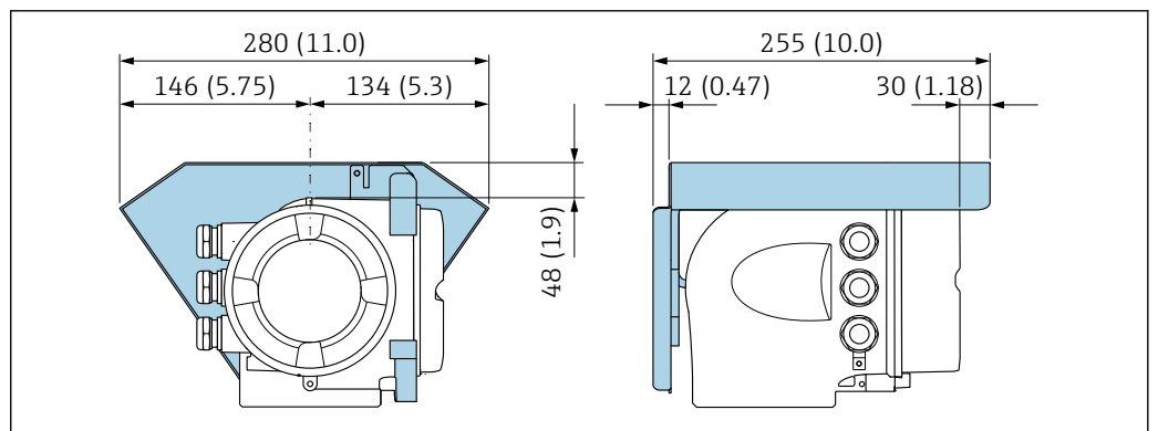
20 Tampa de proteção contra tempo para Proline 500 - unidade mm (pol.)
