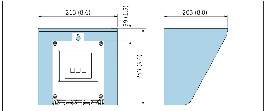
19 Tampa de proteção contra tempo para Proline 500 - digital; unidade mm (pol.)
