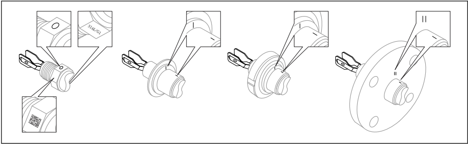
图 13 参照标记水平安装在罐体中的时的音叉位置
