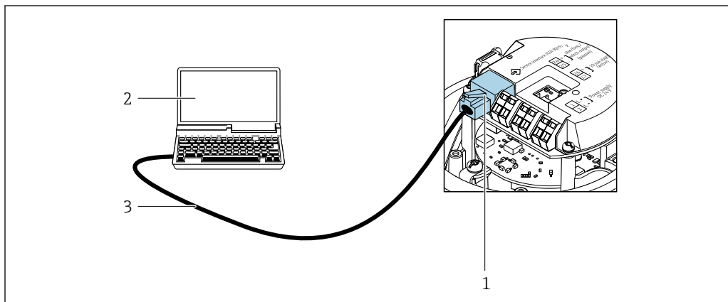
33 Подключение для кода заказа «Выход», опция B «4–20 мА HART, импульсный/частотный/релейный выход»
