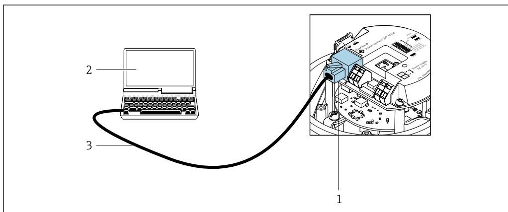
34 Подключение для кода заказа «Выход», опция L «PROFIBUS DP»
