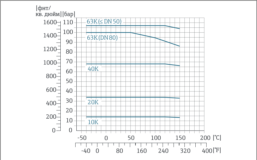
19 С материалом фланца 1.4404 (F316/F316L)
