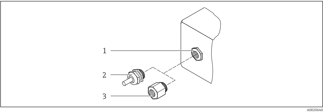
28 Возможные варианты кабельных вводов / кабельных уплотнений
