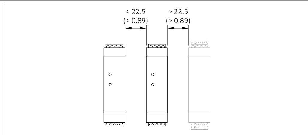
15 Минимальное расстояние до дополнительного искробезопасного защитного барьера Promass 100 или других блоков. Единица измерения, мм (дюйм). Единица измерения – мм (дюйм)
