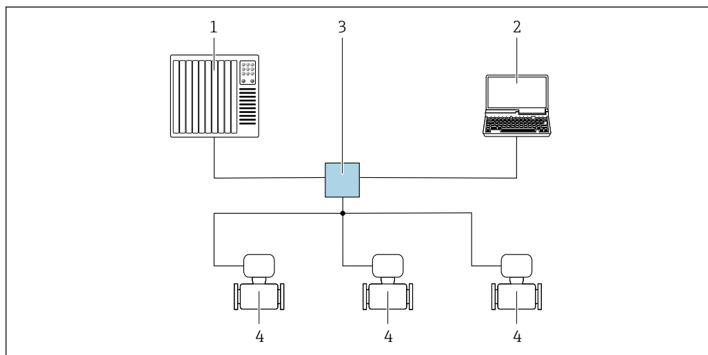
32 Варианты дистанционного управления через сеть PROFINET: топология «звезда»
