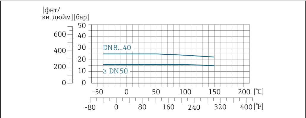
20 С материалом фланца 1.4404 (316/316L)
