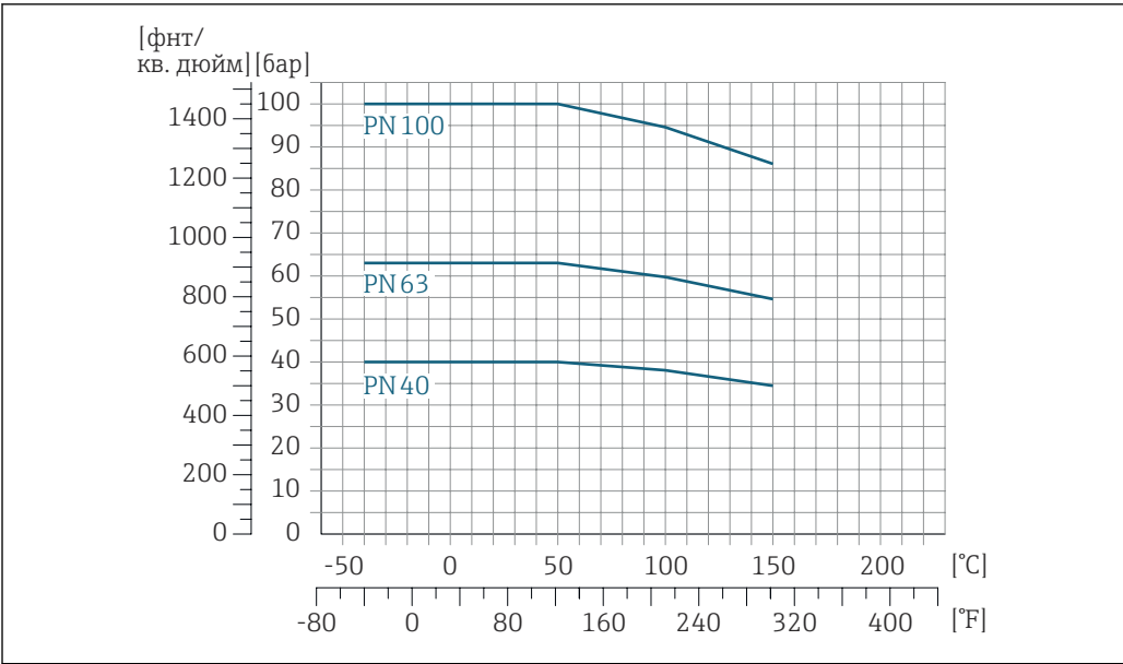
17 С материалом фланца 1.4404 (F316/F316L)
