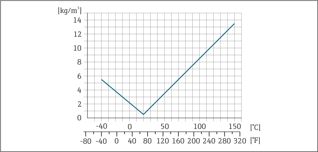
12 Калибровка по плотности на месте эксплуатации, в примере при +20 °C (+68 °F)
