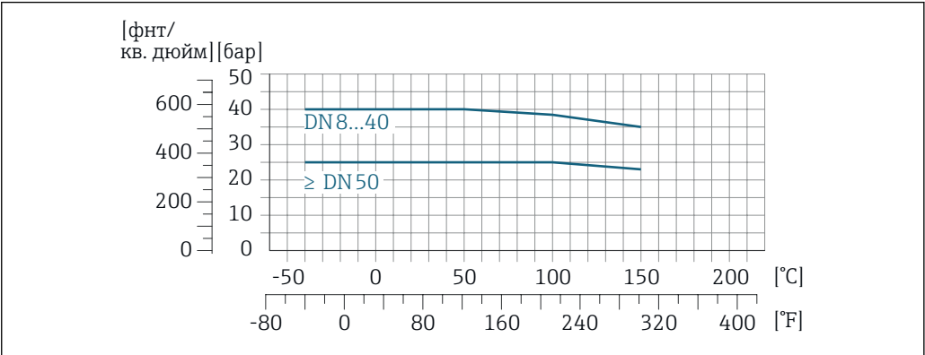
21 С материалом присоединения 1.4404 (316/316L)
