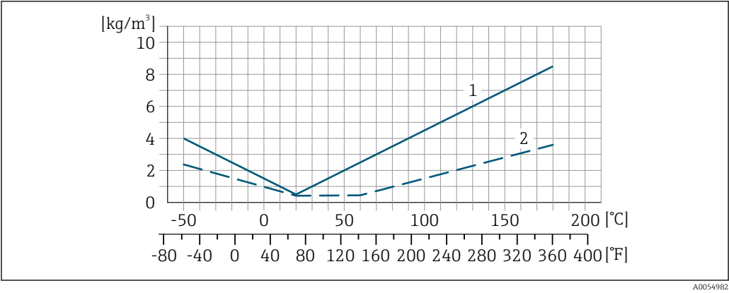
1 Калибровка по плотности на месте эксплуатации, в примере при +20 °C (+68 °F) 2 Расширенная калибровка плотности
