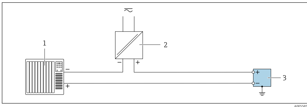
22 Пример подключения для релейного выхода
