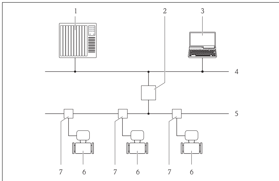
13 Opções para operação remota através da rede PROFIBUS PA
