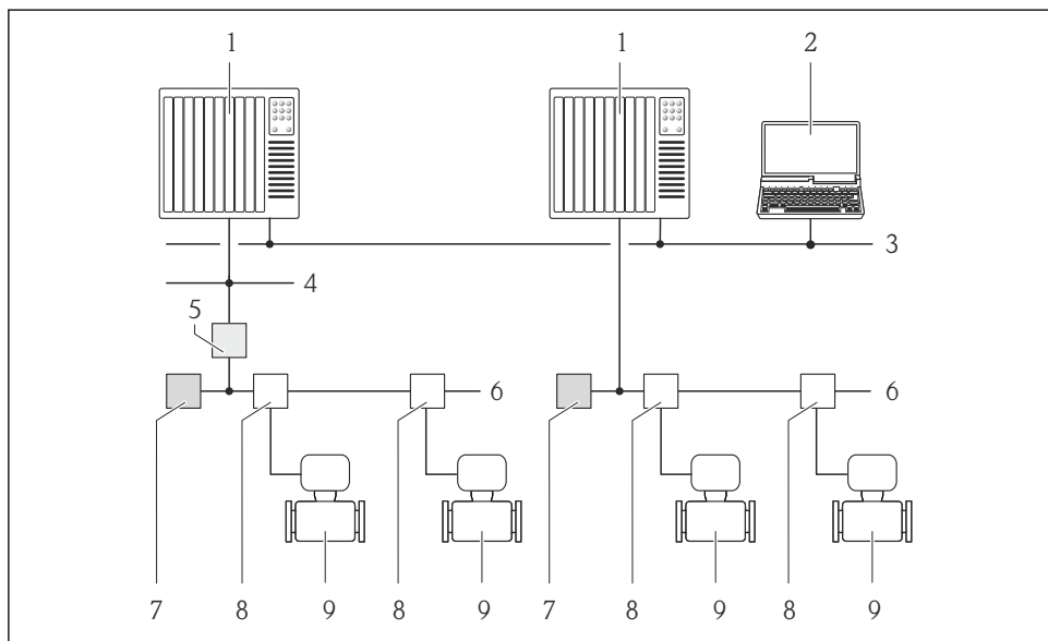
12 Opções para operação remota através da rede FOUNDATION Fieldbus
