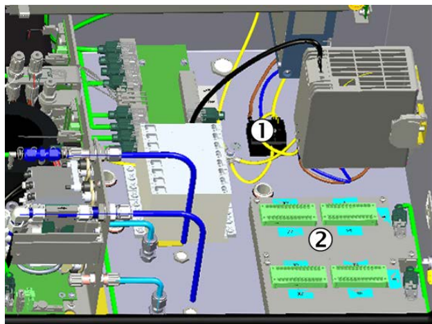
rys. 4: Przyłącza elektryczne
