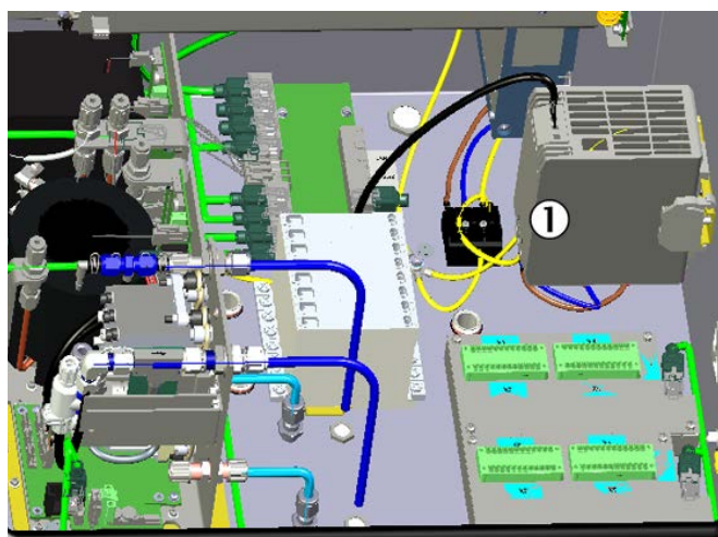
rys. 7: zasilacz
