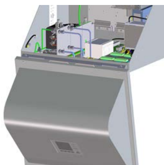
rys. 8: Wwieszona pokrywa
