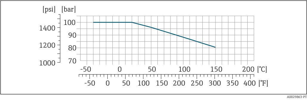
31 Com material da conexão: 1.4404 (316/316)
