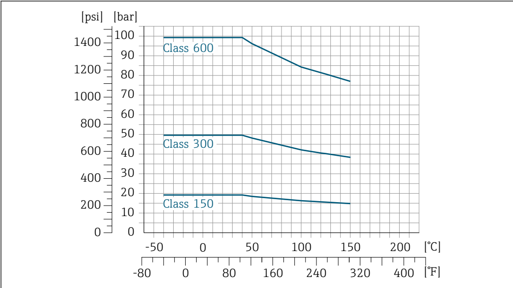
24 Com material do flange 1.4404 (F316/F316L)
