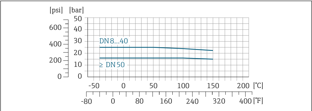
26 Com material do flange 1.4404 (316/316L)
