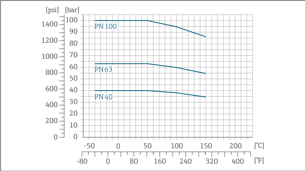
23 Com material do flange 1.4404 (F316/F316L)
