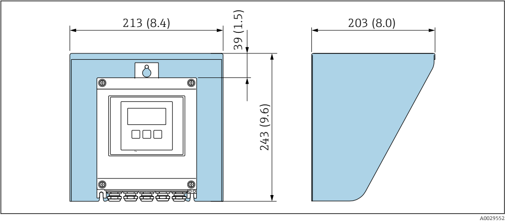
20 Tampa de proteção contra tempo para Proline 500 - digital; unidade mm (pol.)
