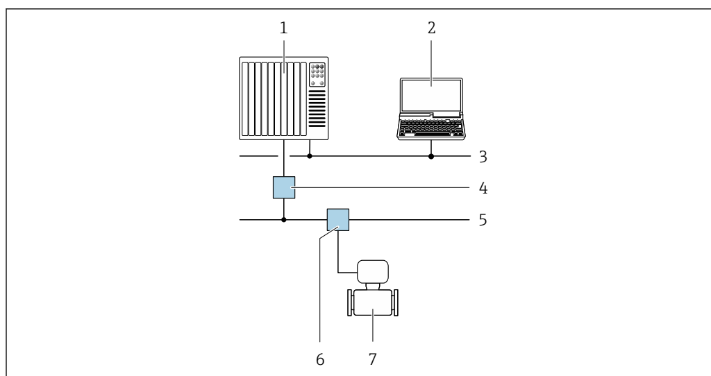
52 Opções para operação remota através da rede PROFIBUS PA
