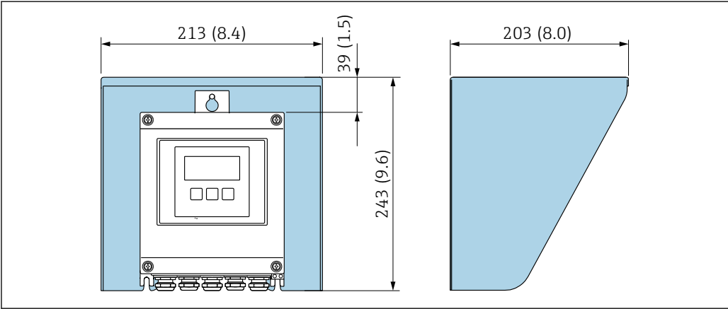
40 Tampa de proteção contra tempo para Proline 500 - digital; unidade mm (pol.)
