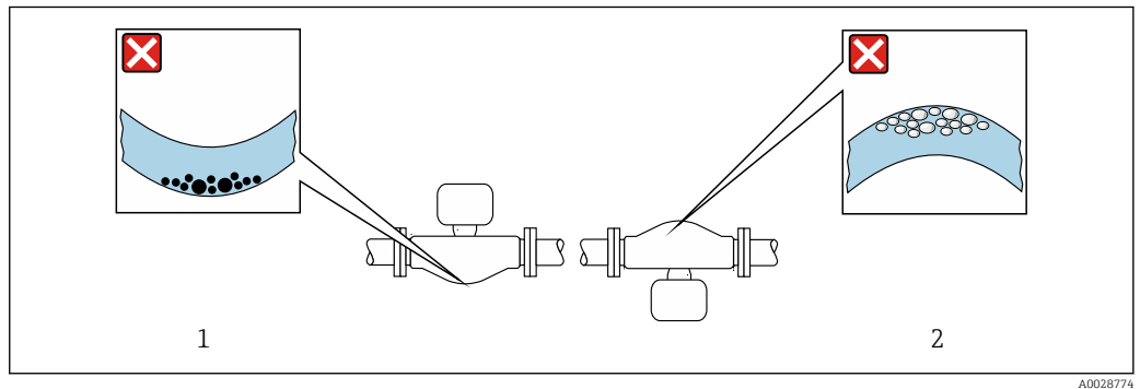
15 Direção do sensor com tubo de medição curvado
