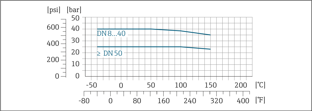
27 Com material da conexão: 1.4404 (316/316)
