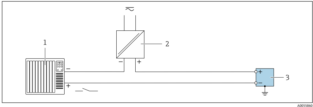
图 25 状态输入
