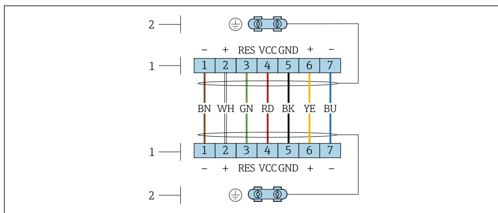
4 Morsetti per vano connessioni nel supporto da parete del trasmettitore e nella custodia di connessione del sensore
