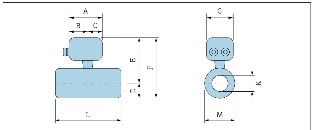
Versione con saldatura di testa secondo ASME: Classe 600/900/1500, Scheda 80/160
