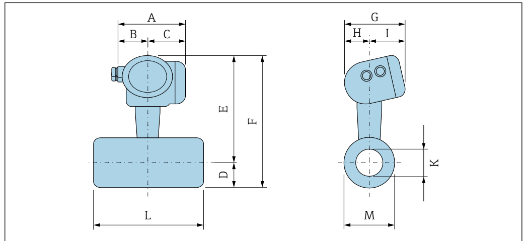
Versione con saldatura di testa secondo ASME: Classe 600/900/1500, Scheda 80/160 Codice d'ordine per "Connessione al processo", opzione A6B/A6C
