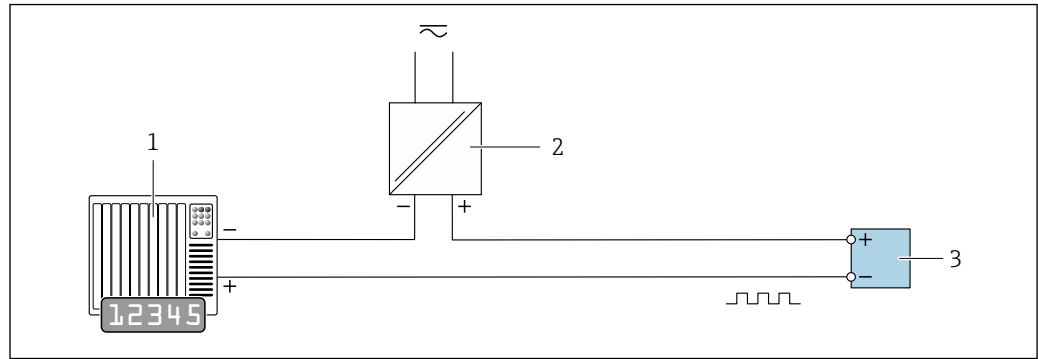
4 Anschlussbeispiel für Impuls-/Frequenz Ausgang (passiv)
