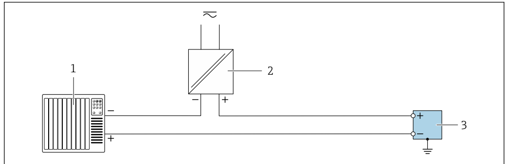
☑ 9 接线实例：脉冲输出/频率输出/开关量输出（无源）
