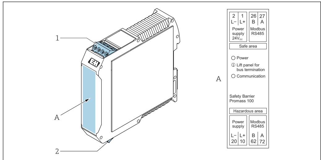
图 8 Promass 100 安全栅，带接线端子 1 非防爆危险区、Zone 2, Cl. I, Div. 2 防爆危险区 2 本安防爆区
