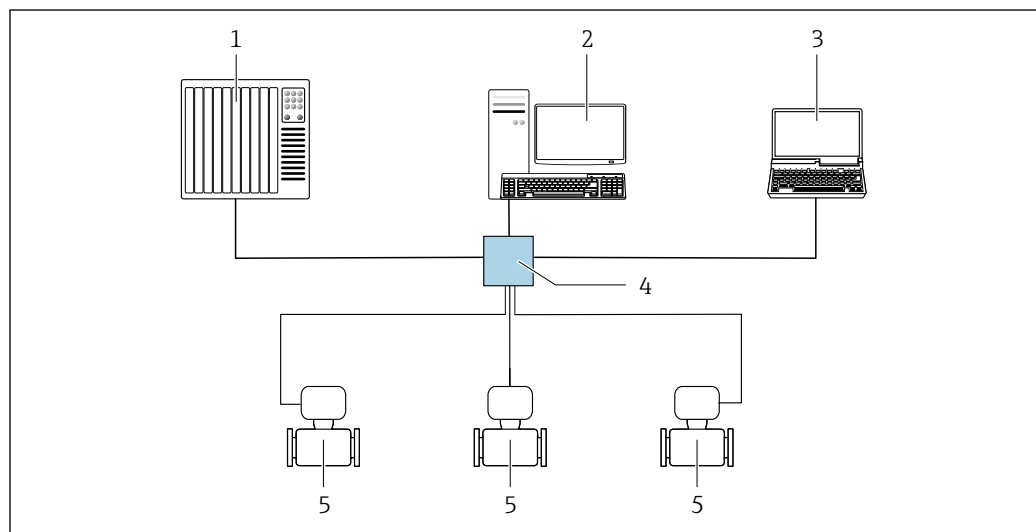
图 35 通过 EtherNet/IP 网络进行远程操作：星形拓扑结构
