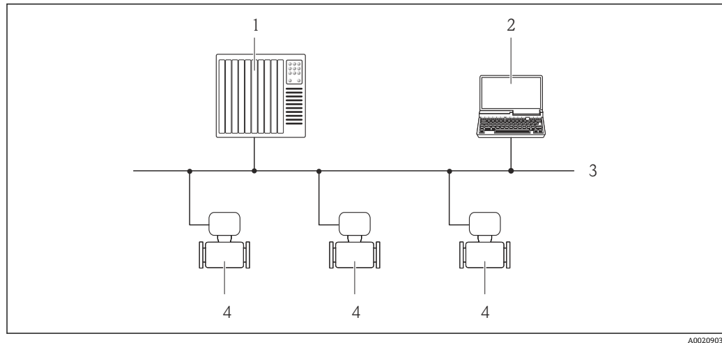
图 34 通过 PROFIBUS DP 网络进行远程操作
