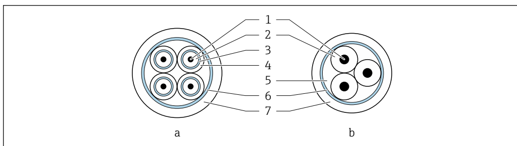
图 8 电缆截面图
