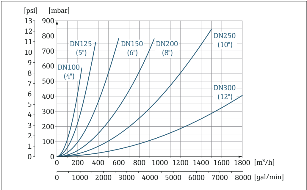
19 压损：适用口径 DN 100...300 (4...12"); 订购选项“设计”，选型代号 C “固定法兰，缩径测量管，无前后直管段长度要求”
