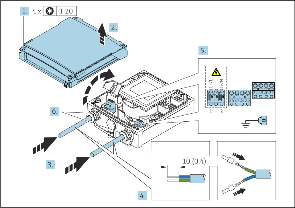
图 14 连接电源
