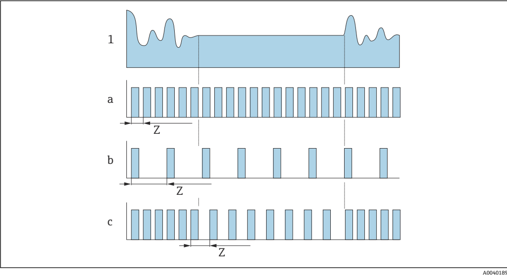
16 不同数据记录方式的工作原理 1 曲线图 a 最小测量间隔时间（外接电源） b 固定测量间隔时间：介于传感器相关最小值和 60 秒之间 c 智能适应 Z 测量间隔时间
