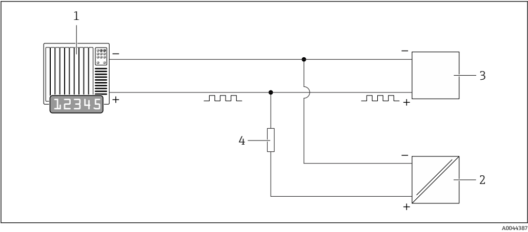
15 接线实例：脉冲输出（无源信号） 1 自动化系统，带脉冲输入（例如 PLC） 2 外接直流电源（例如 24 VDC 电源） 3 变送器的集电极开路脉冲输入：注意输入参数→ 92 4 上拉电阻（例如 10 kΩ）
