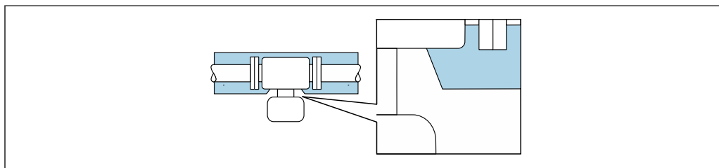
31 Aislamiento térmico con cuello de extensión expuesto
