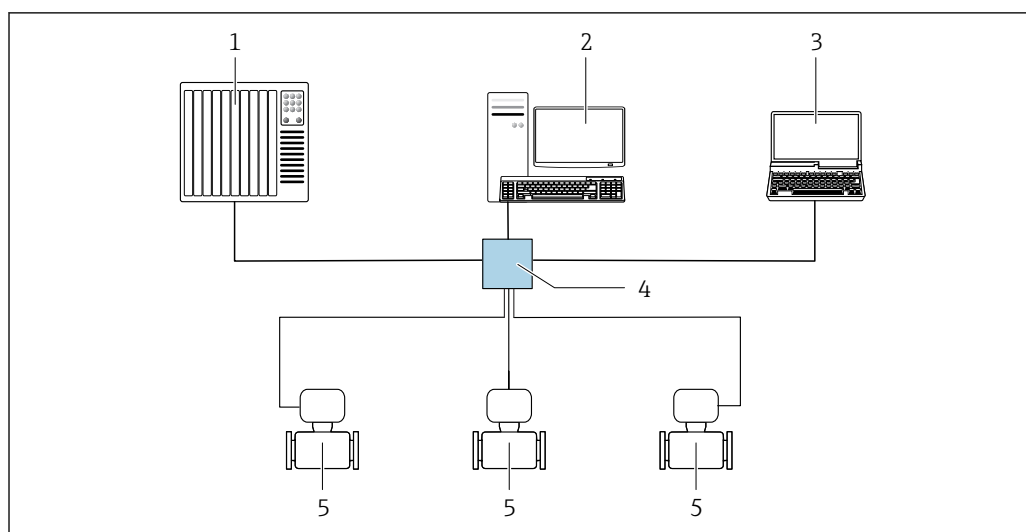
図 49 EtherNet/IP ネットワーク経由のリモート操作オプション：スター型トポロジー
