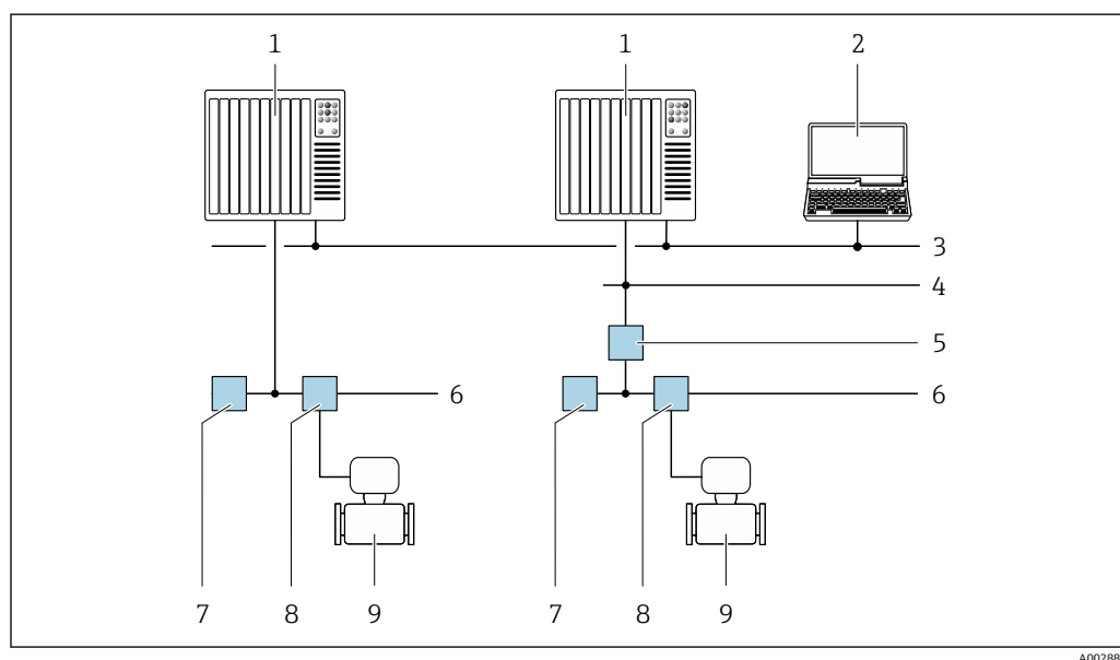
45 FOUNDATION Fieldbus ネットワークを介したリモート操作のオプション
