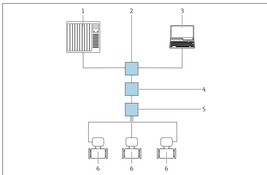
図 53 Modbus TCP over Ethernet-APL プロトコル経由のリモート操作用オプション (アクティブ)
