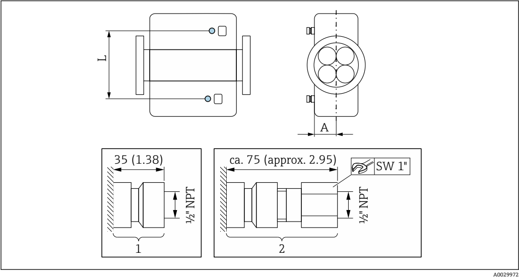
34 1 パージ接続用の接続ニップル：「センサオプション」のオーダーコード、オプション CH「パージ接続」 2 破裂板付き接続ニップル：「センサオプション」のオーダーコード、オプション CA「破裂板」
