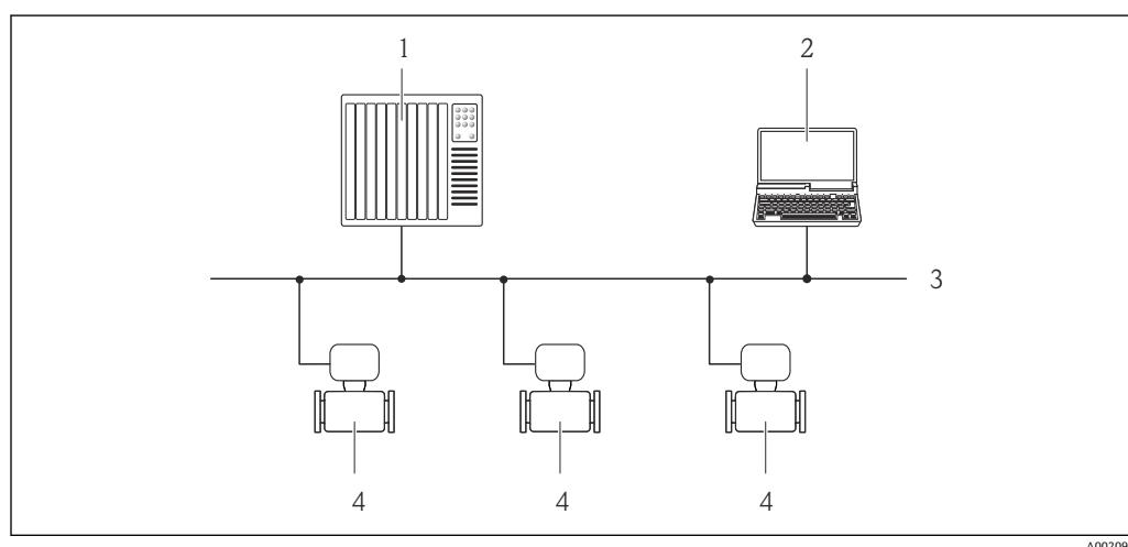
46 PROFIBUS DP ネットワークを介したリモート操作のオプション
