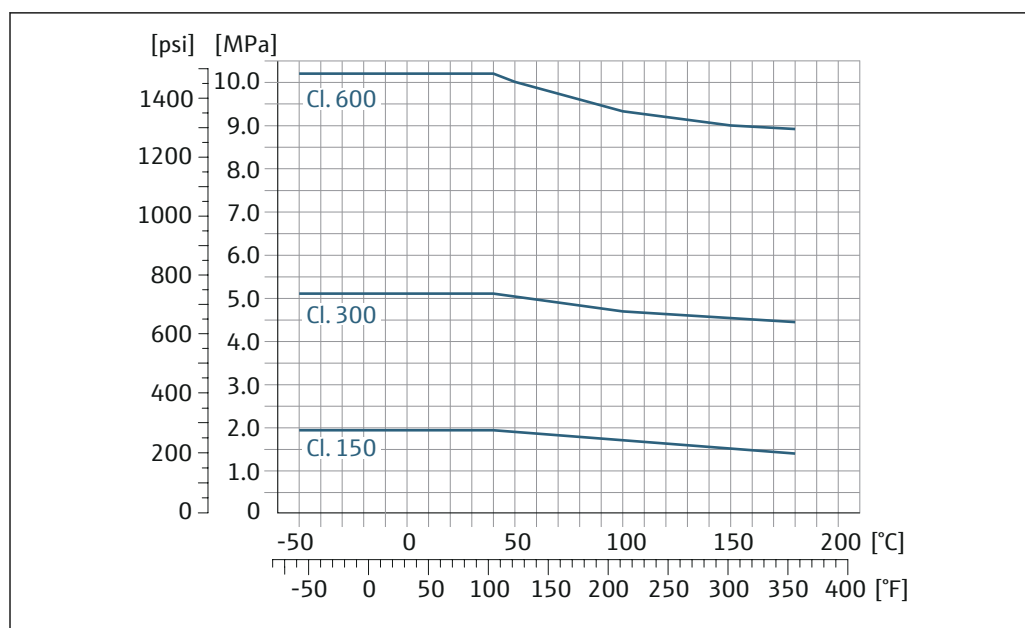
図 23 フランジ材質 1.4404 (SUS 316 相当または SUS 316L 相当)
