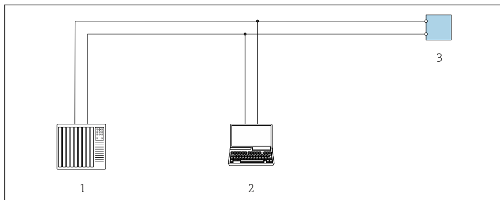
図 48 Modbus RS485 プロトコル経由のリモート操作オプション（アクティブ）
