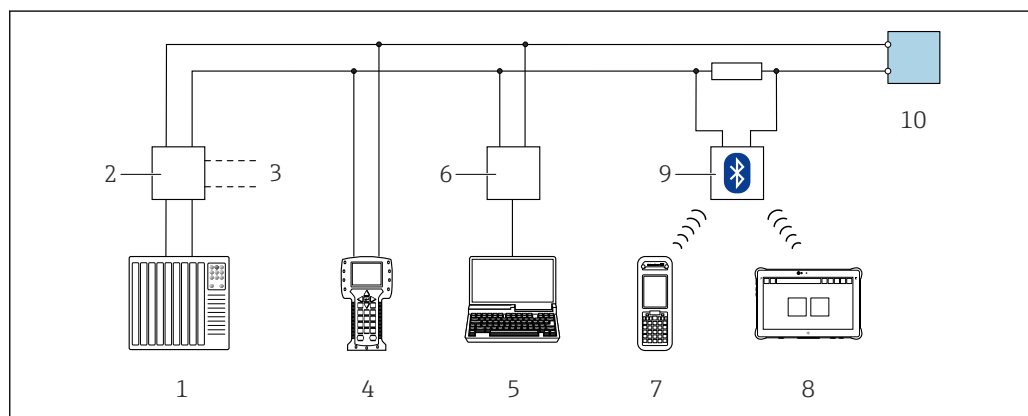
図 44 HART プロトコル経由のリモート操作オプション（パッシブ）
