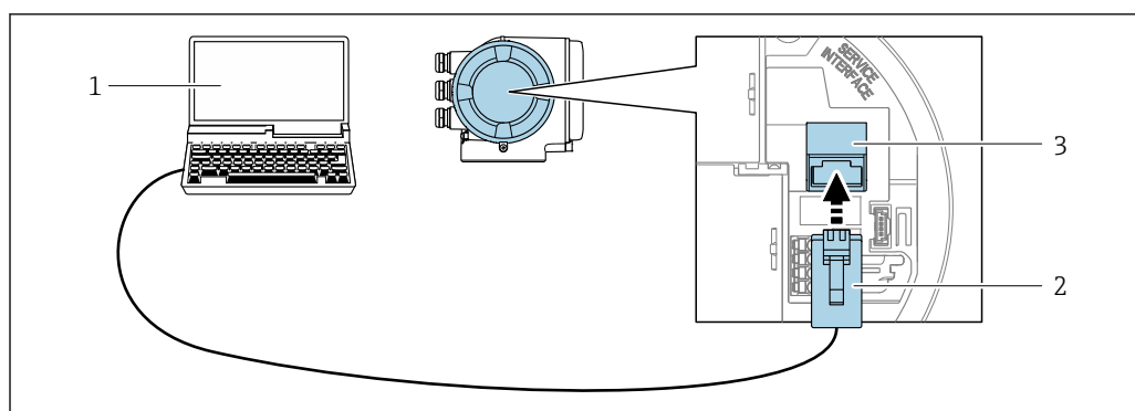
図 56 サービスインタフェース (CDI-RJ45) 経由の接続
