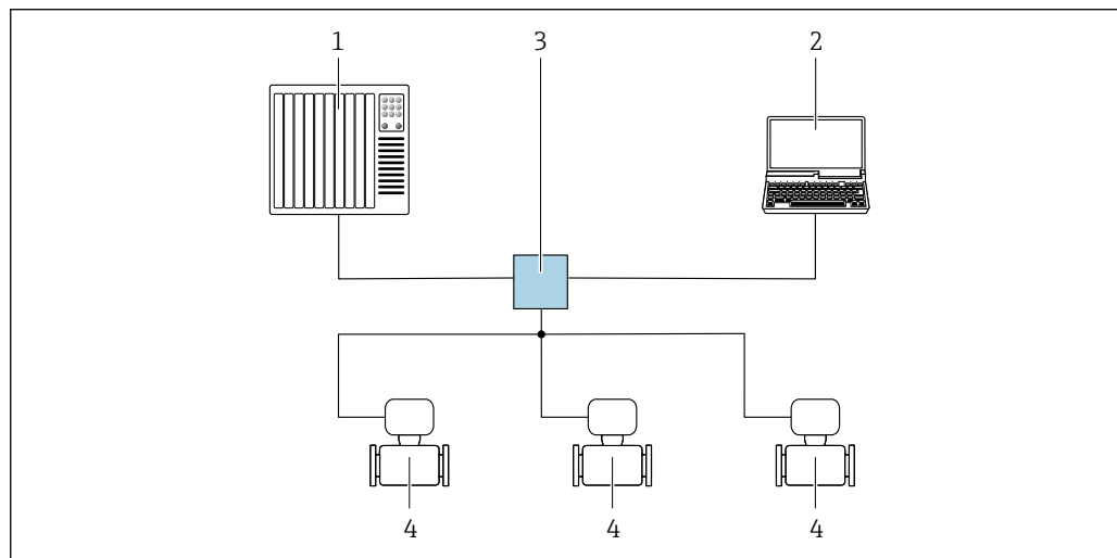
図 51 PROFINET ネットワーク経由のリモート操作オプション：スター型トポロジー
