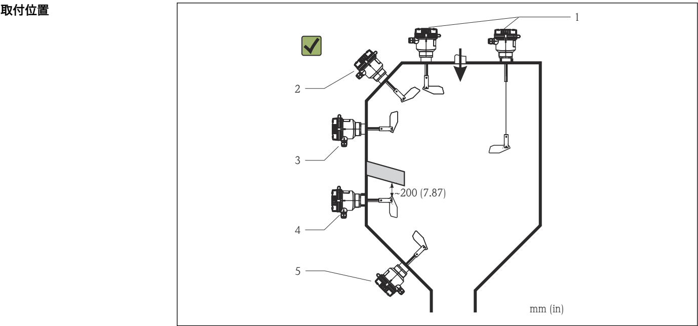
図 3 許容される機器の取付位置
