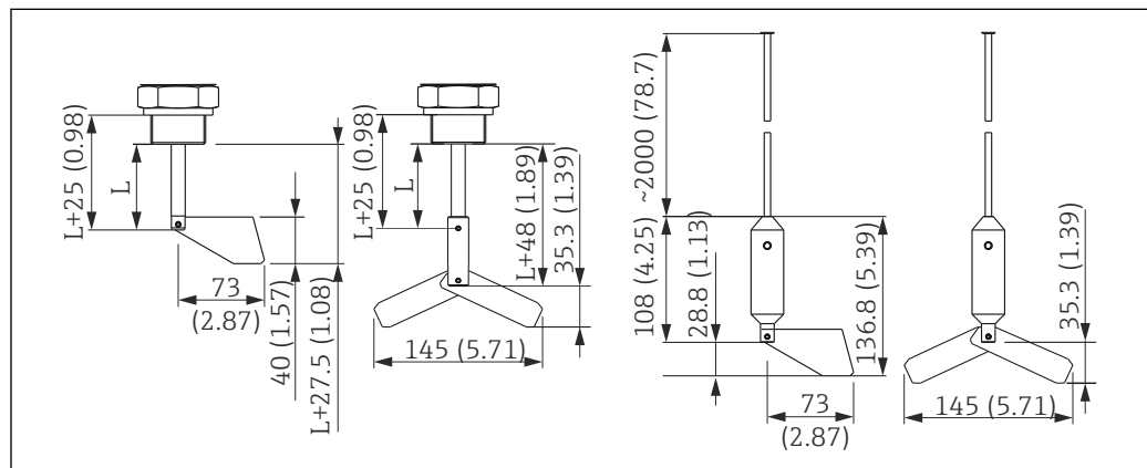
図 6 回転パドルの寸法 - 標準/ヒンジ、シャフト/伸長ロープ用 (単位 mm (in))
