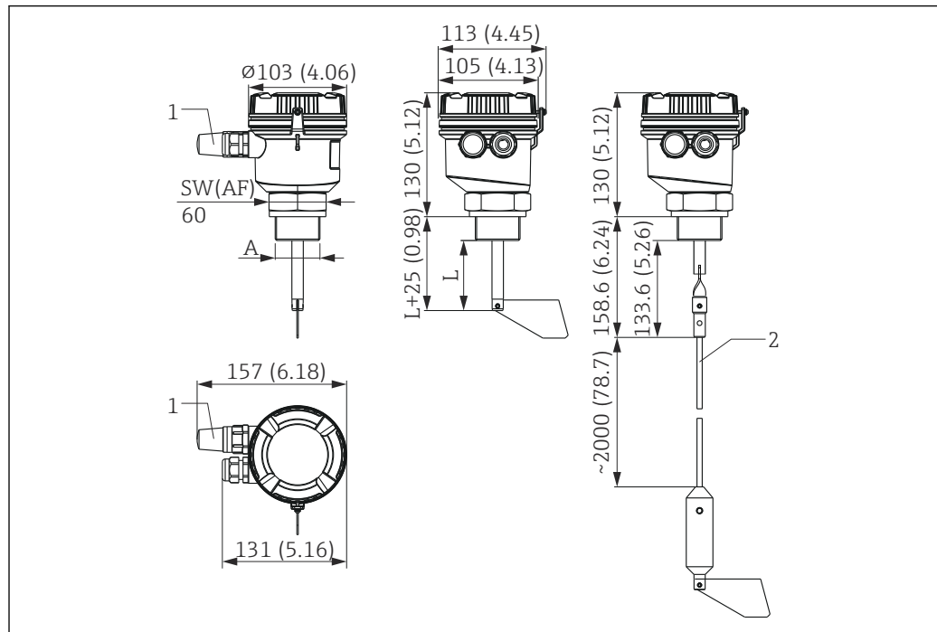
図 5 レベルスイッチの寸法 (単位 mm (in))
