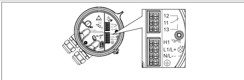
図 2 レベルスイッチの端子の割当て
