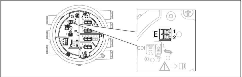
图 36 NMS8x 的接线端子，用于连接 NMT81
