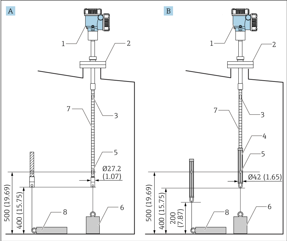
图 28 使用锚固配重。测量单位 mm (in)
