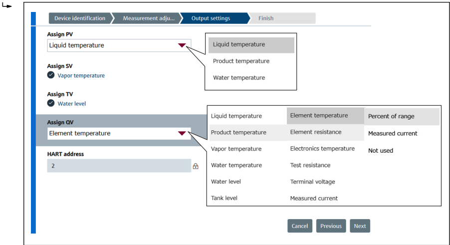
图 47 输出设置界面
