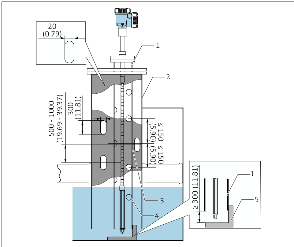
图 30 安装在导波管中。测量单位 mm (in)
