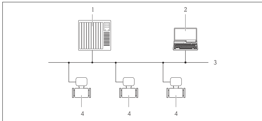
22 Possibilités de configuration à distance via réseau PROFIBUS DP
