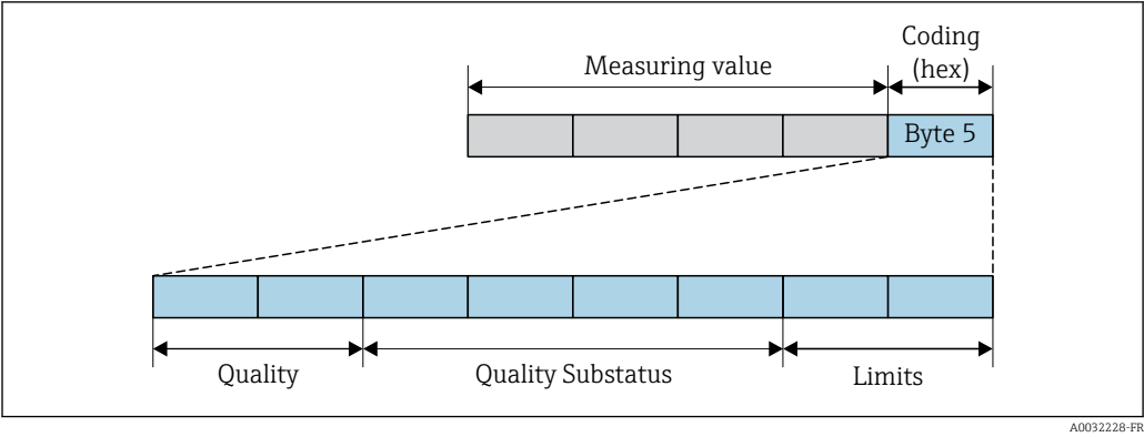
29 Structure de l'octet de codage
