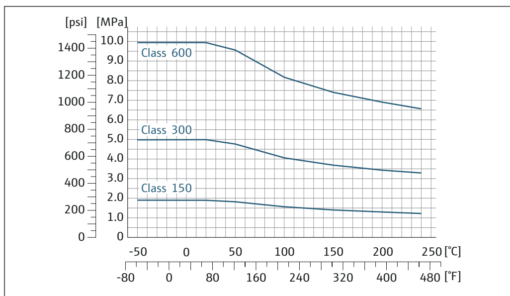
図 21 フランジ材質 1.4301 (SUS F304 相当) ; 接液部 アロイ C22
