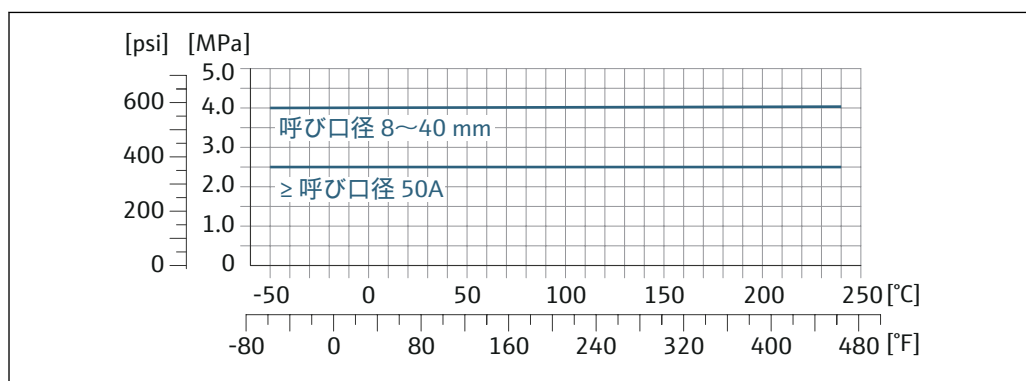
図 23 接続部の材質 1.4404 (SUS 316 または 316L 相当)
