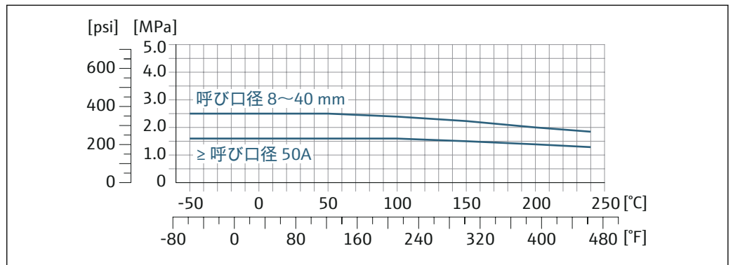
図 19 接続部の材質 1.4404 (SUS 316 または 316L 相当)
