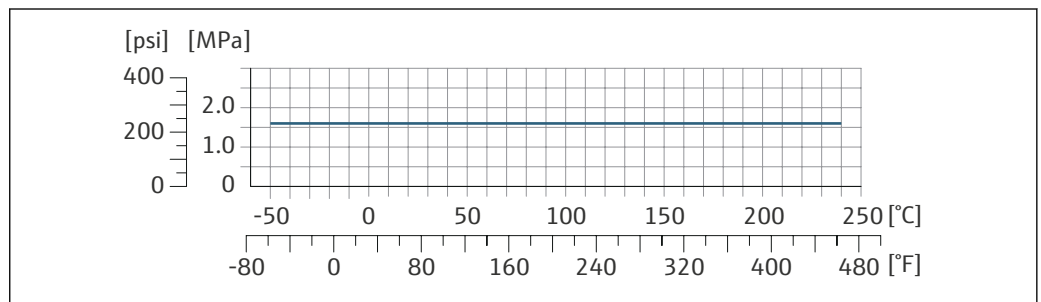
図 26 接続部の材質 1.4404 (SUS 316 または 316L 相当)
