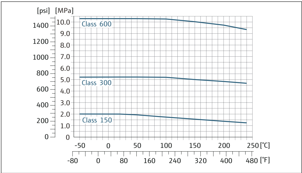
図 17 フランジ材質 アロイ C22
