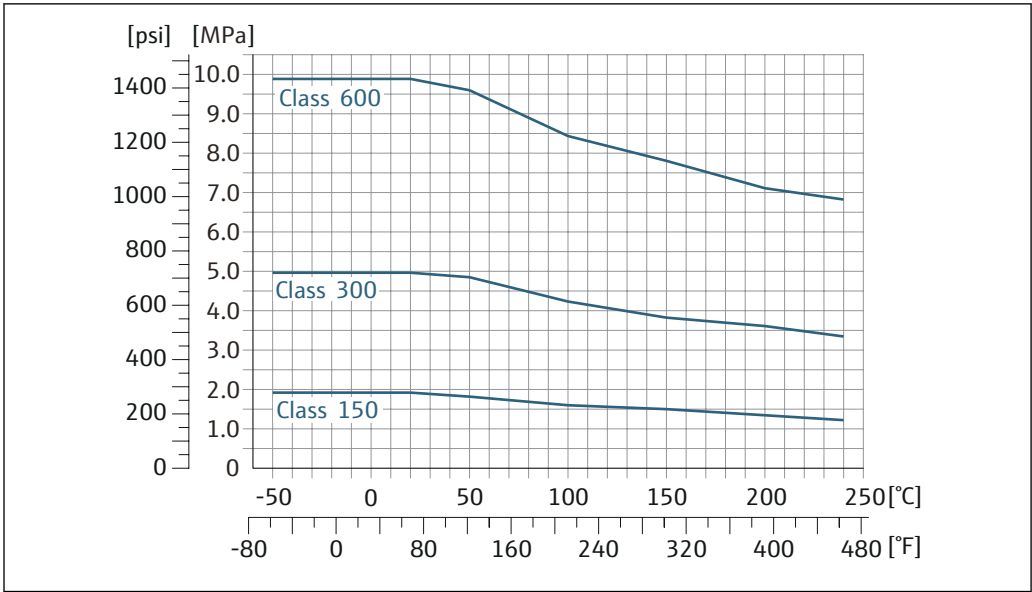
図 16 フランジ材質 1.4404 (SUS F316 または F316L 相当)
