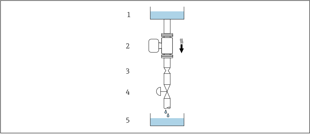
図 12 下り配管への設置（例：バッチアプリケーション用）
