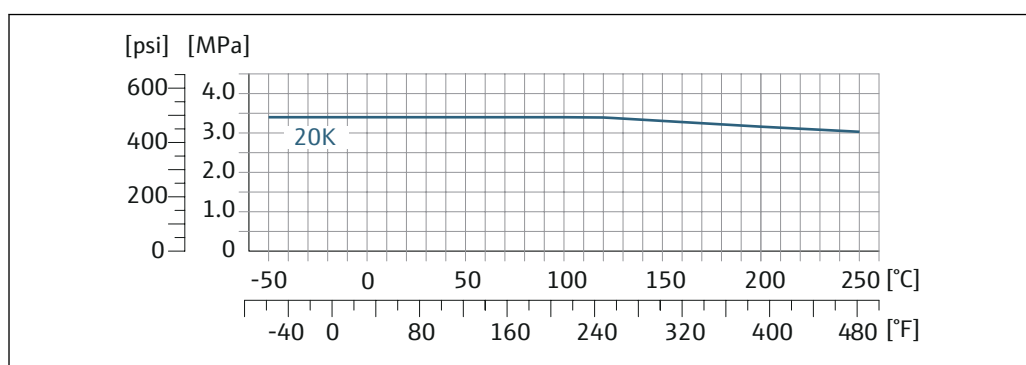
図 22 フランジ材質 1.4301 (SUS F304 相当) ; 接液部 アロイ C22
