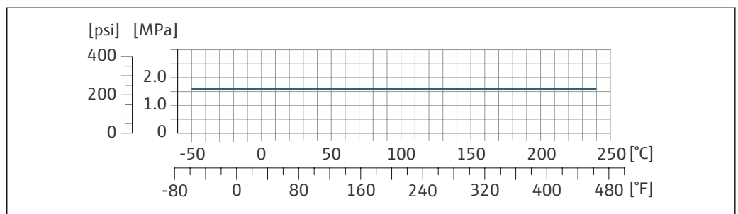
図 25 接続部の材質 1.4404 (SUS 316 または 316L 相当)
