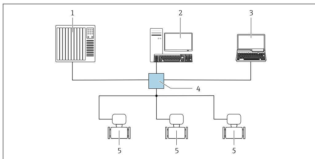
図 34 EtherNet/IP ネットワーク経由のリモート操作オプション：スター型トポロジー
