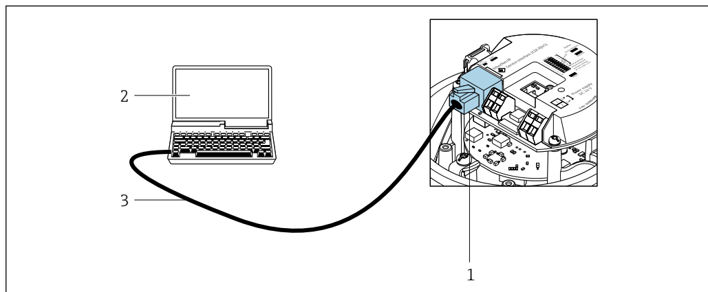
図 37 「出力」のオーダーコードの接続、オプション L : PROFIBUS DP
