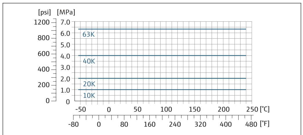
図 18 フランジ材質 1.4404 (SUS F316 または F316L 相当)、アロイ C22
