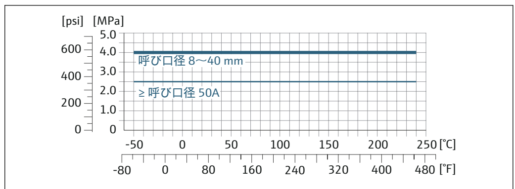
図 24 接続部の材質 1.4404 (SUS 316 または 316L 相当)
