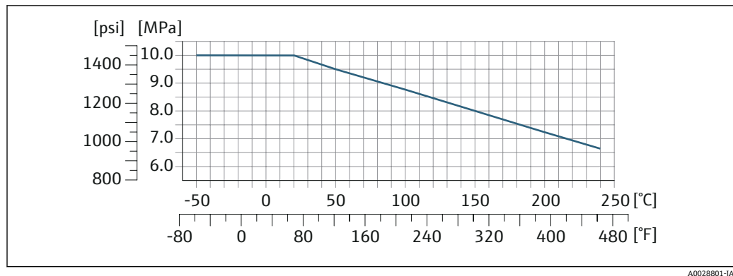
図 27 接続部の材質 1.4404 (SUS 316 または 316L 相当)
