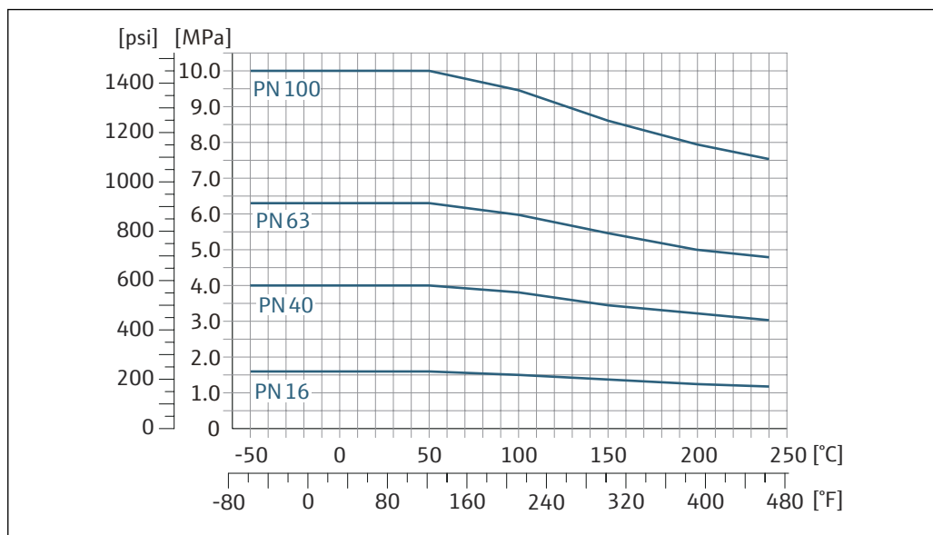
図 15 フランジ材質 1.4404 (SUS F316 または F316L 相当)、アロイ C22
