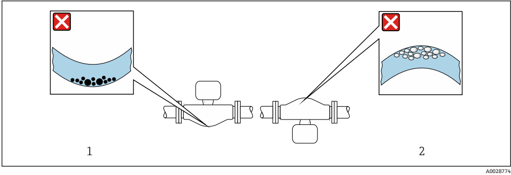
☑ 13 弓形計測チューブセンサの取付方向
