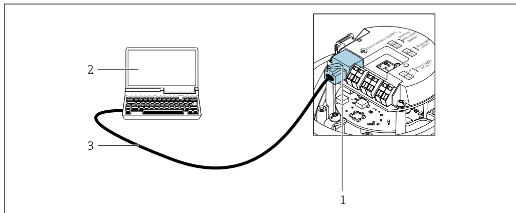
図 36 「出力」のオーダーコードの接続、オプション B : 4~20 mA HART、パルス/周波数/スイッチ出力
