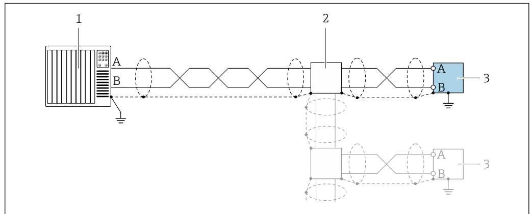
25 Пример подключения для Modbus RS485
