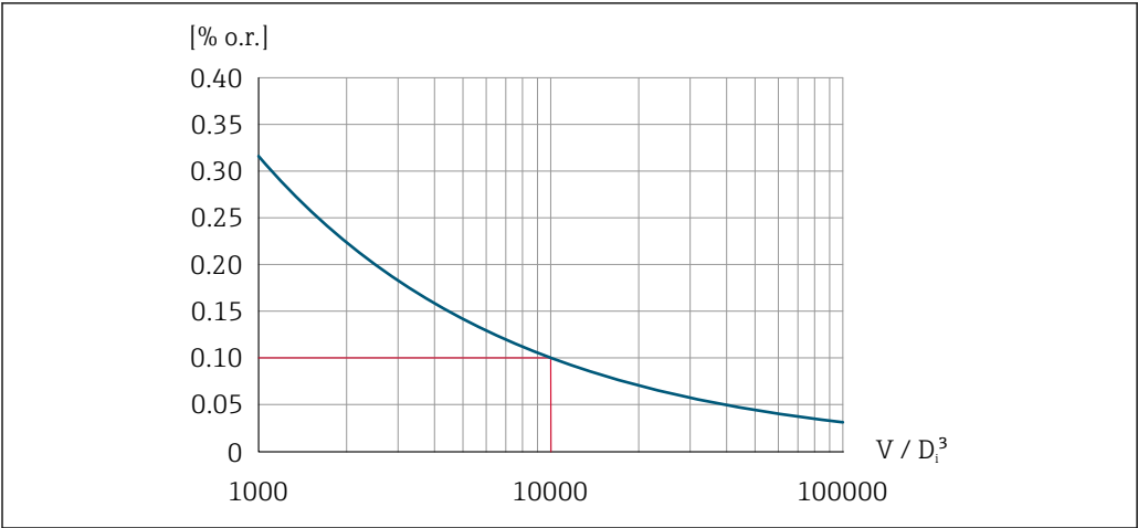
27 Повторяемость – 0,1 % ИЗМ при измерении объемного расхода (м³) от V = 10\,000 \cdot D_i^3
