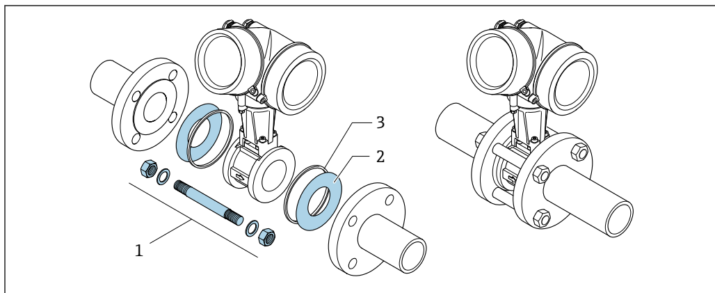
7 Монтажный комплект для бесфланцевого исполнения
