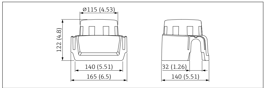
23 Wetterschutzhaube für Einkammergehäuse Aluminium. Maßeinheit mm (in)
