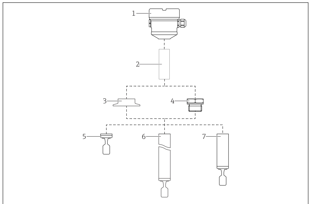
2 Produktaufbau Liquiphant FTL63
