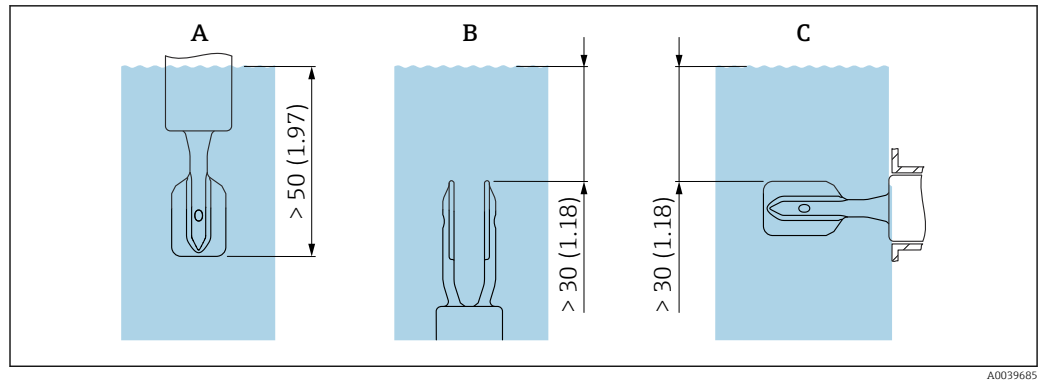
5 Maßeinheit mm (in)
