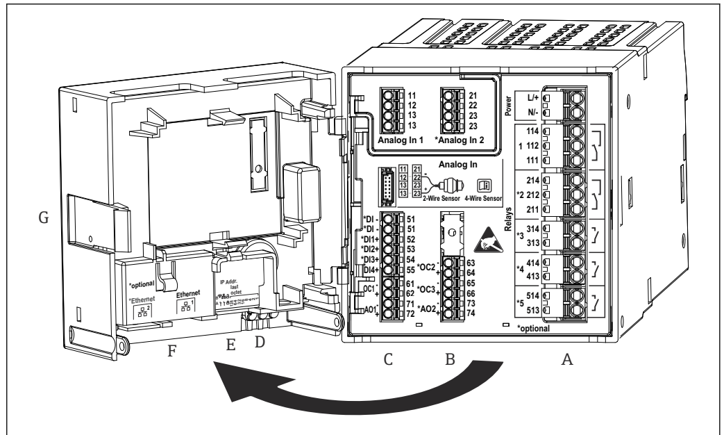
42 Anschlussklemmen Hutschienengerät; Klemmenausführung: steckbare Push-in-Klemmen
