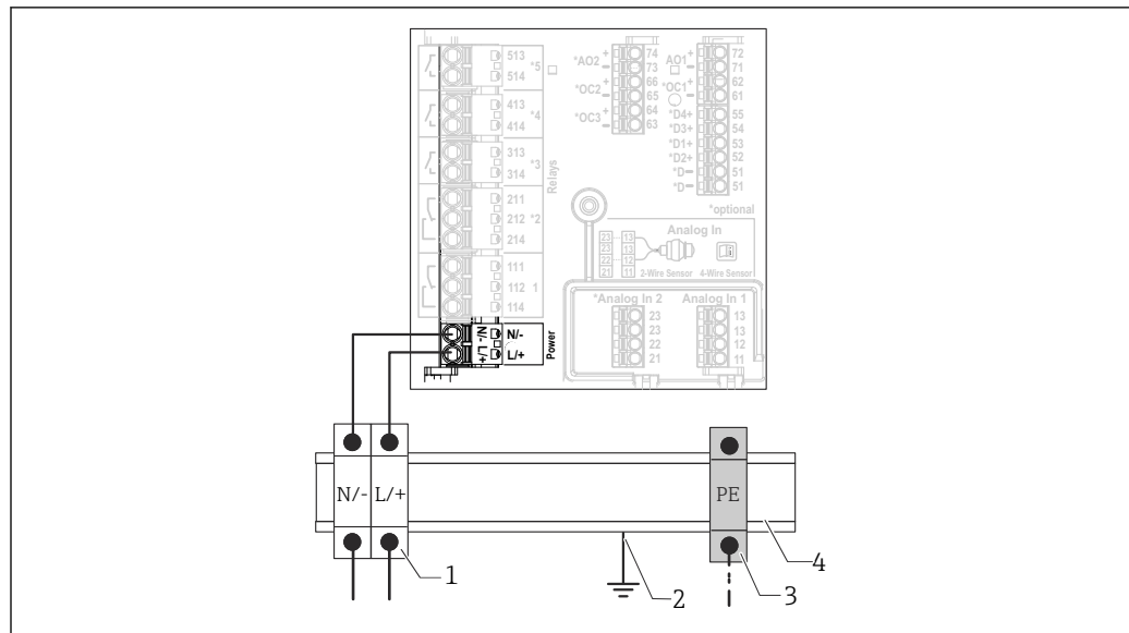
27 Anschluss Hilfsenergie am Schalttafelgerät
