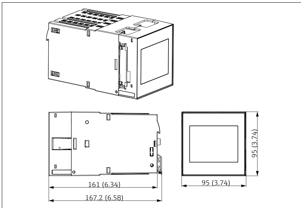
11 Abmessungen Hutschienengerät. Maßeinheit mm (in)
