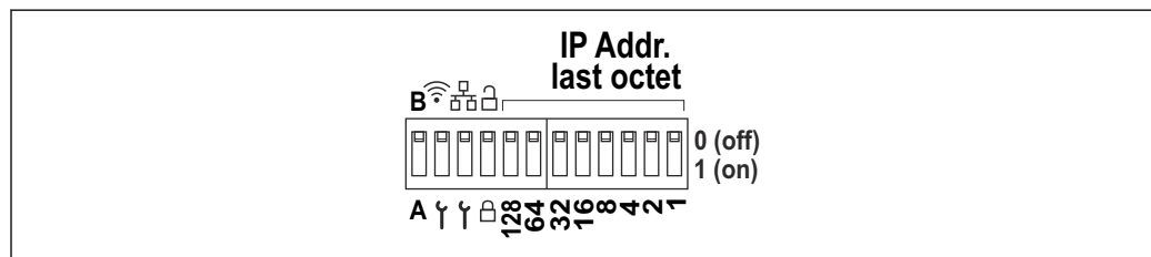
28 DIP-Schalter (Zeichnung zeigt den Auslieferungszustand)
