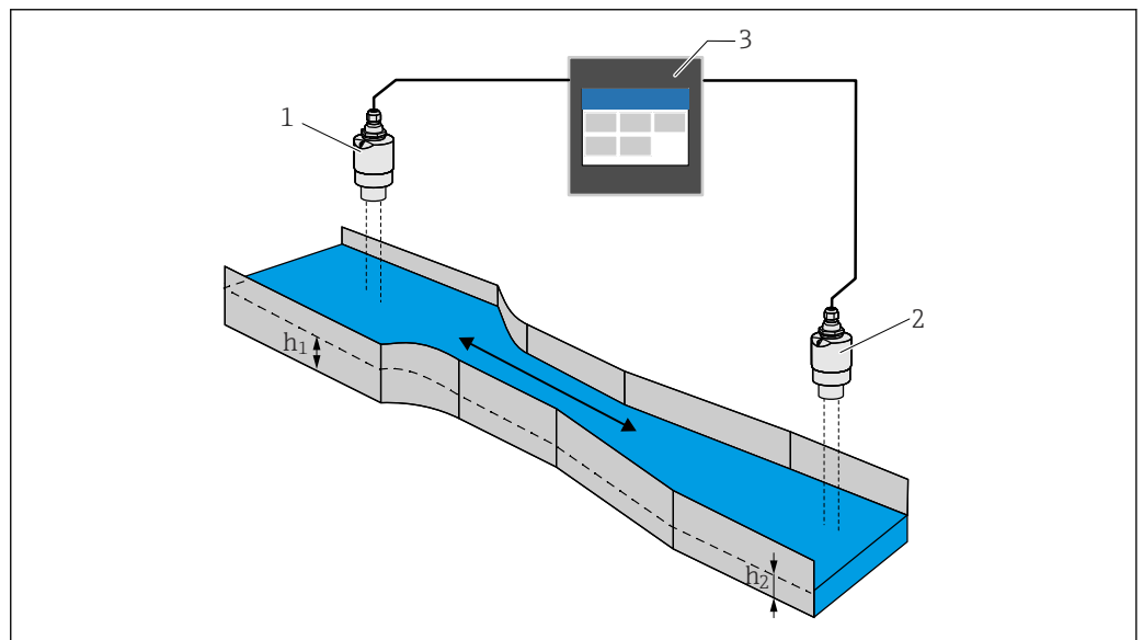
36 Rückstauerkennung
