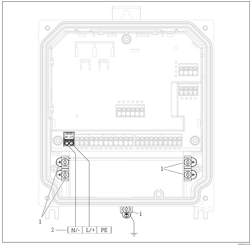
24 Anschluss Hilfsenergie im Feldgehäuse Polycarbonat
