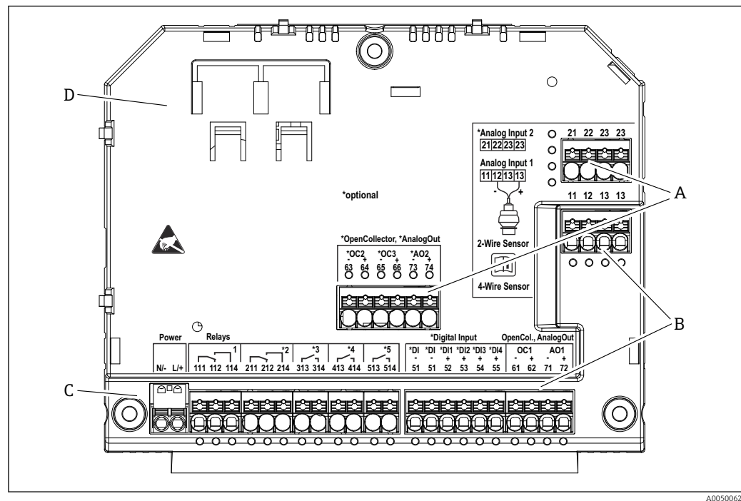
20 Anschlussklemmen im Klemmenraum Feldgehäuse Polycarbonat; Klemmenausführung: Push-in-Klemmen
