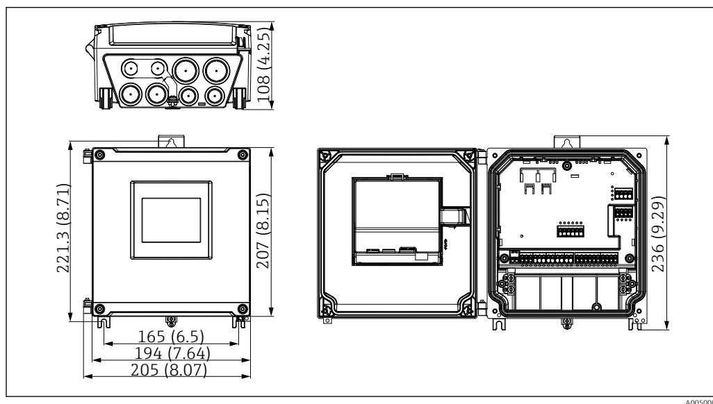
5 Abmessungen Feldgehäuse Polycarbonat. Maßeinheit mm (in)
