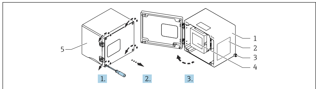
16 Zugang zum Klemmenraum im Feldgehäuse Aluminium
