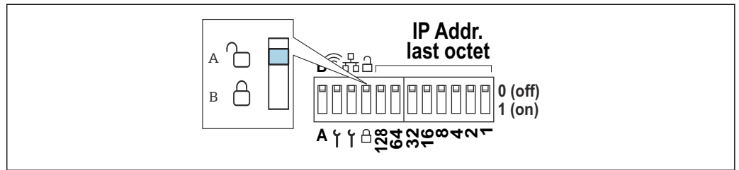
39 Hardware-Verriegelung per DIP-Schalter
