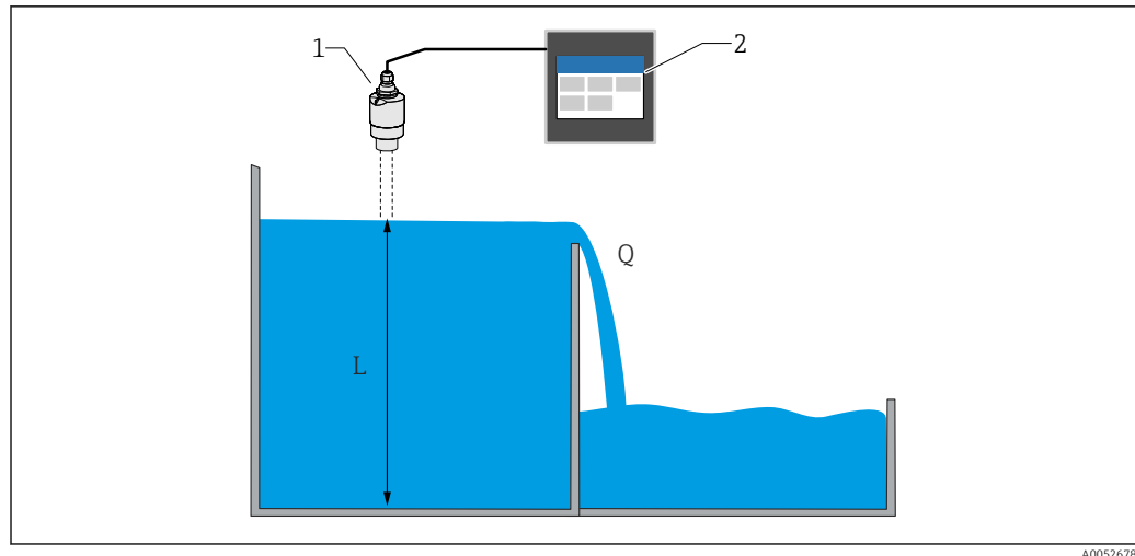
37 Regenüberlaufbecken
