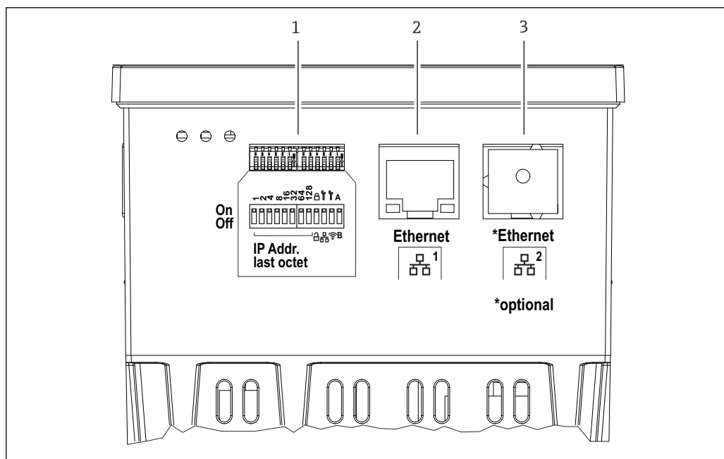
44 Anschlüsse Schalttafelgerät (Geräteunterseite)
