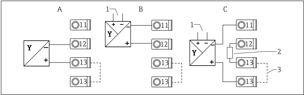
23 Anschlussbeispiele 2-Leiter- und 4-Leiter Sensor am 4 ... 20 mA Stromeingang bzw. HART
