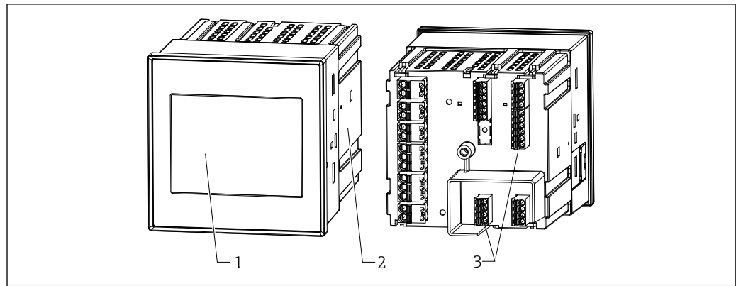
4 Aufbau Schalttafelgerät
