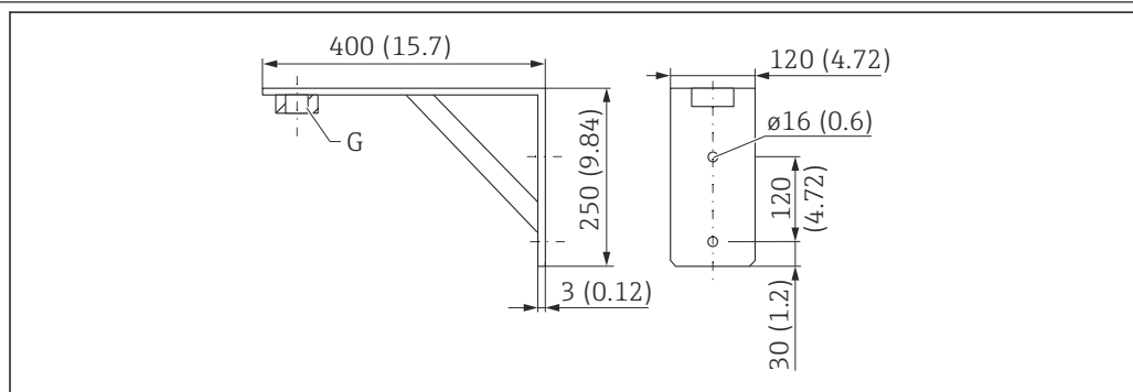
41 Dimensões do suporte de montagem. Unidade de medida mm (in)
