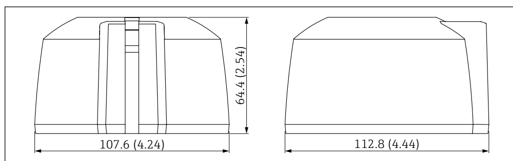
29 Dimensões da tampa de proteção G1/NPT1, entrada para cabos por cima. Unidade de medida mm (in)
