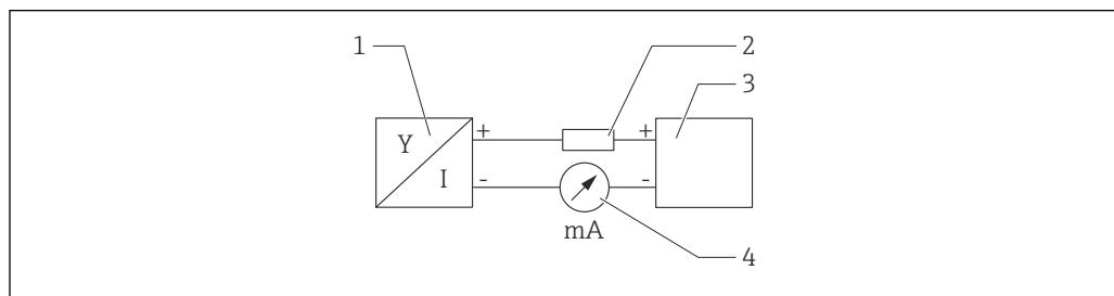
4 Diagrama de função da conexão HART
