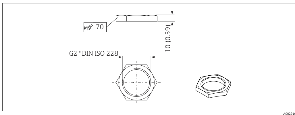
32 Dimensões da porca de fixação. Unidade de medida mm (in)
