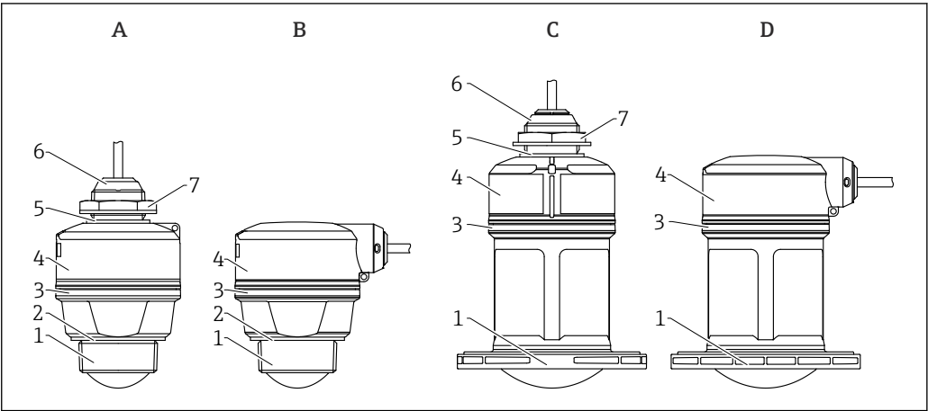
26 Projeto do instrumento
