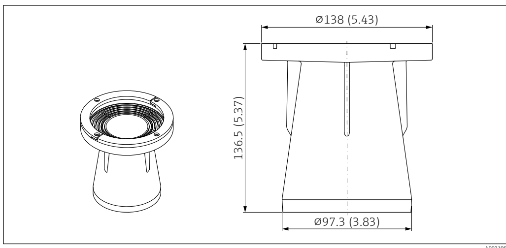
36 Dimensões do tubo de proteção contra transbordamento 80 mm (3 in). Unidade de medida mm (in)
