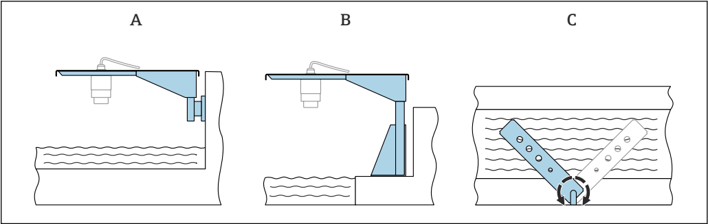
18 Instalação escorada, com pivô
