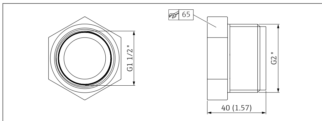
33 Dimensões do adaptador Uni
