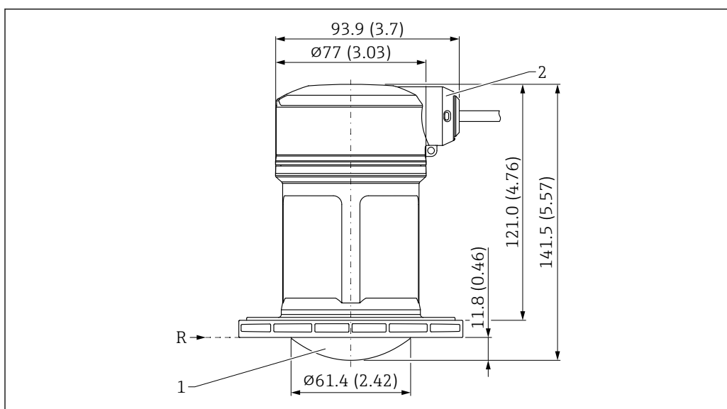
24 Dimensões; antena 80 mm (3 in) com entrada para cabo na lateral
