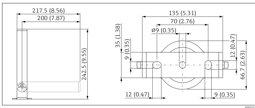
40 Dimensões do suporte de montagem. Unidade de medida mm (in)
