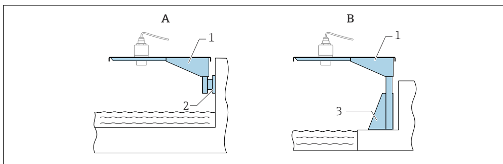
45 Tipo de instalação da conexão de processo na extremidade da antena do sensor
