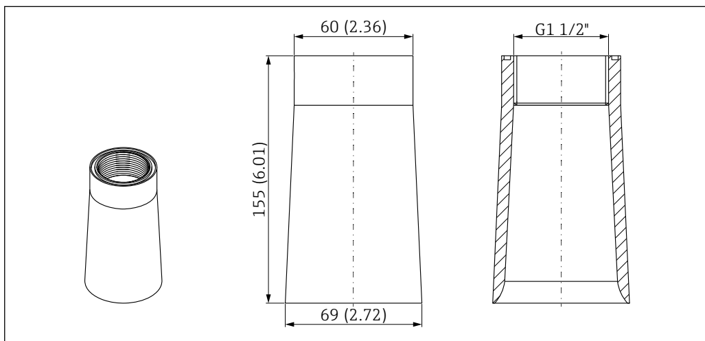
35 Dimensões do tubo de proteção contra transbordamento 40 mm (1.5 in). Unidade de medida mm (in)
