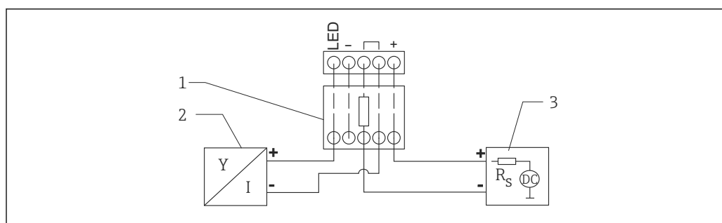
8 Diagrama de função do equipamento HART, RIA15 com iluminação, módulo de resistor de comunicação HART
