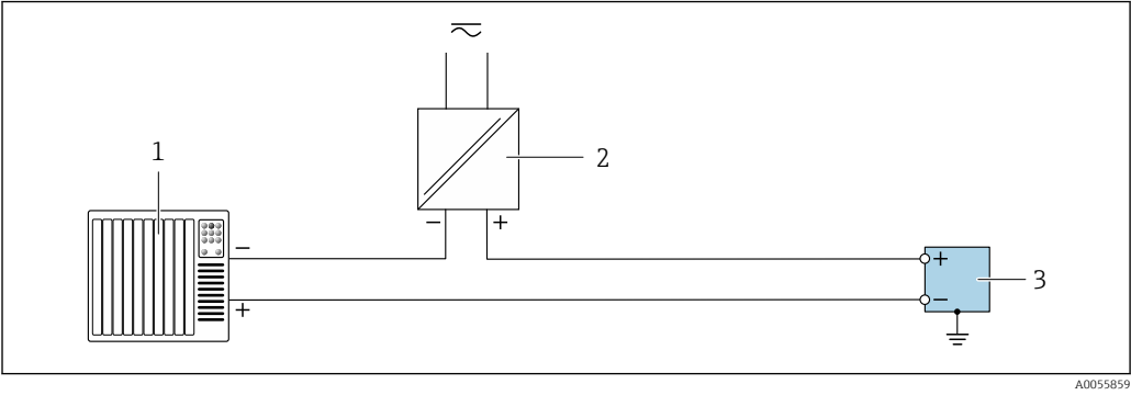
23 Ejemplo de conexión para salida de relé 1 Sistema de automatización con entrada de conmutación (p. ej., PLC) 2 Alimentación 3 Transmisor con salida de relé
