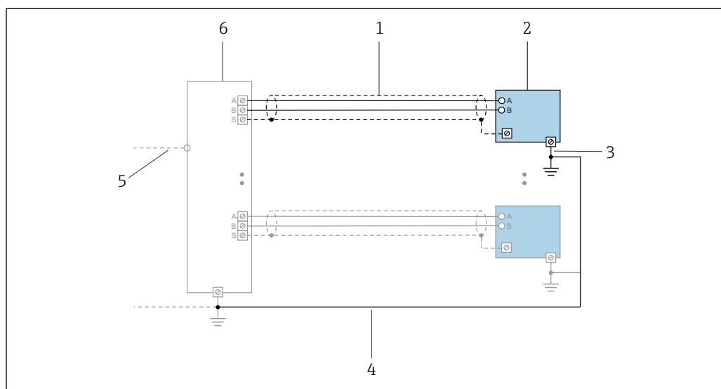
15 Ejemplo de conexión para PROFINET sobre Ethernet-APL
