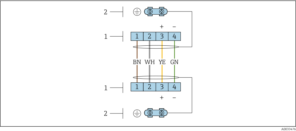
12 Anschlussklemmen für Anschlussraum im Wandhalter des Messumformers und dem Anschlussgehäuse des Messaufnehmers 1 Anschlussklemmen für Verbindungskabel 2 Erdung erfolgt über Kabelzugentlastung
