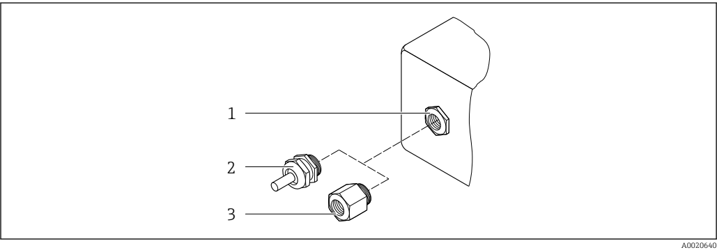
31 Mögliche Kabeleinführungen/-verschraubungen
