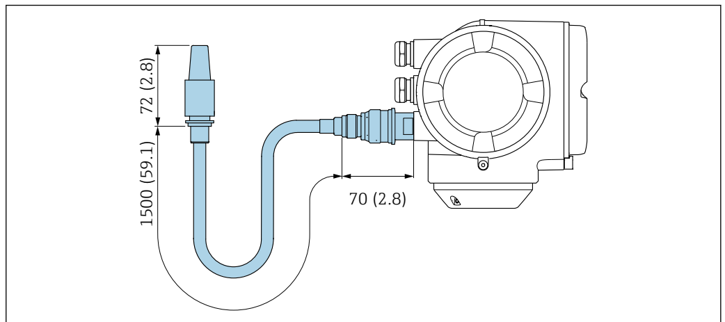
45 Ед. изм.: мм (дюймы)
