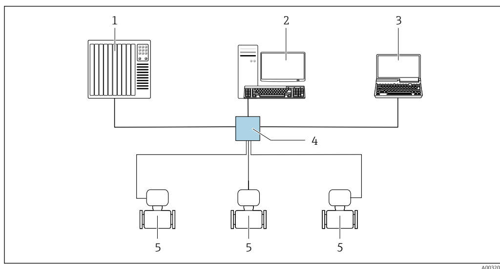
54 Варианты дистанционного управления через сеть EtherNet/IP: топология «звезда»
