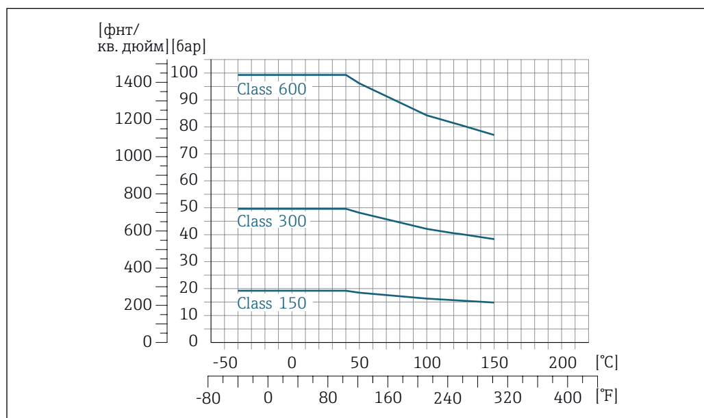
24 С материалом фланца 1.4404 (F316/F316L)
