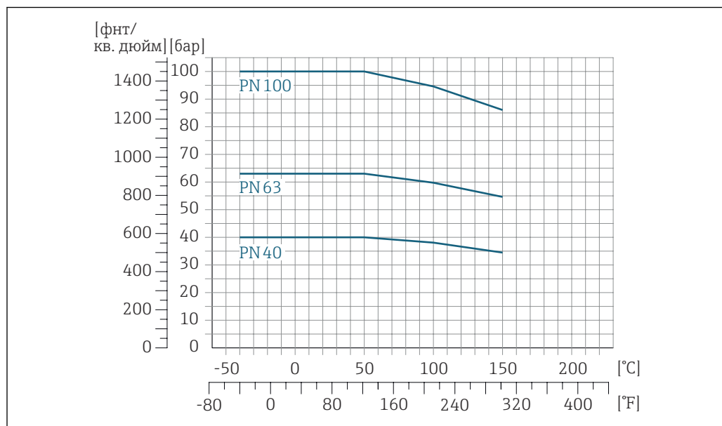
23 С материалом фланца 1.4404 (F316/F316L)
