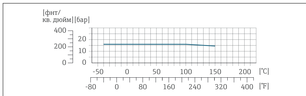
29 С материалом присоединения 1.4404 (316/316L)
