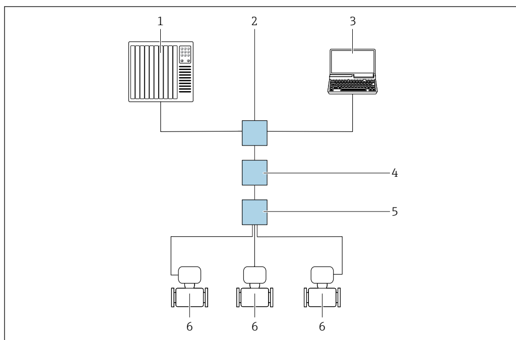
58 Варианты дистанционного управления через протокол Modbus TCP через Ethernet-APL (активный)
