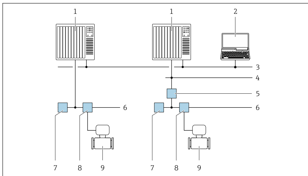
50 Варианты дистанционного управления по сети FOUNDATION Fieldbus
