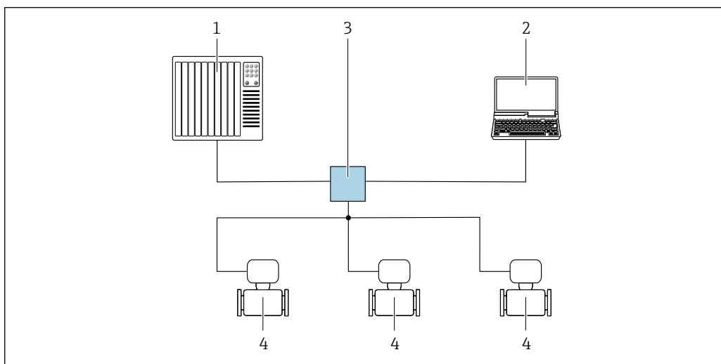
56 Варианты дистанционного управления через сеть PROFINET: топология «звезда»
