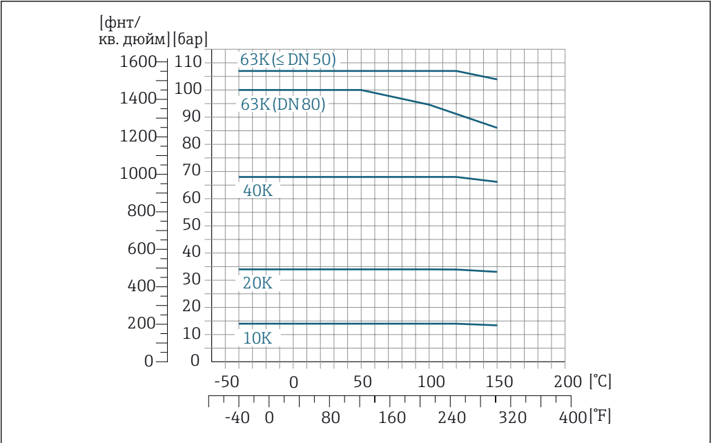
25 С материалом фланца 1.4404 (F316/F316L)
