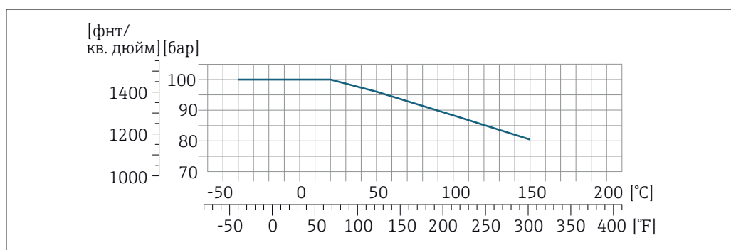
31 С материалом присоединения 1.4404 (316/316L)
