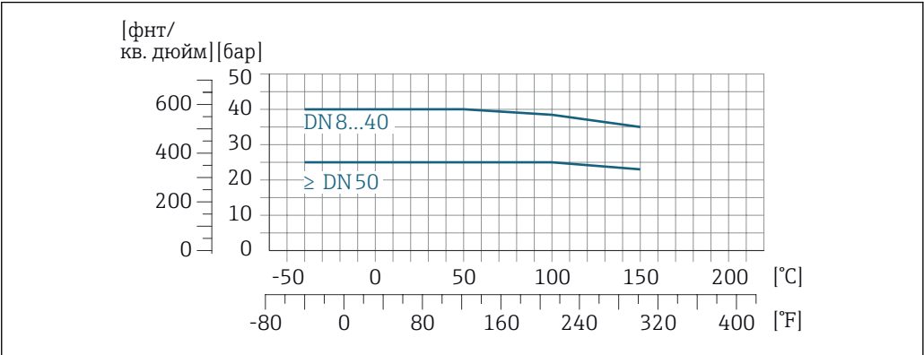
27 С материалом присоединения 1.4404 (316/316L)
