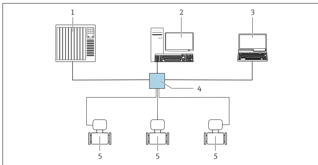
59 Варианты дистанционного управления по протоколу Modbus TCP посредством интерфейса Ethernet - 100 Мбит/с: топология «звезда»
