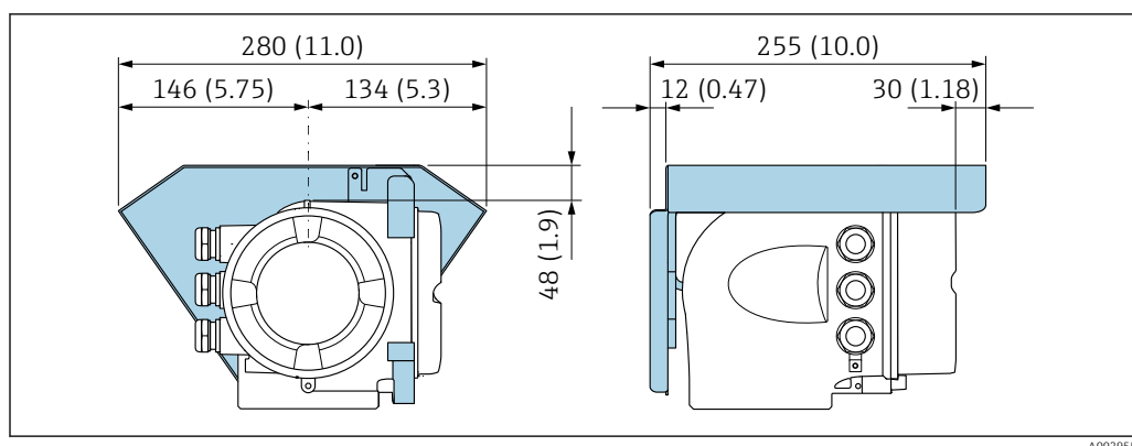
35 Защитный козырек от погодных явлений для Proline 500 – единица измерения- мм (дюймах)
