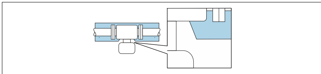
32 Теплоизоляция с открытой удлинительной шейкой
