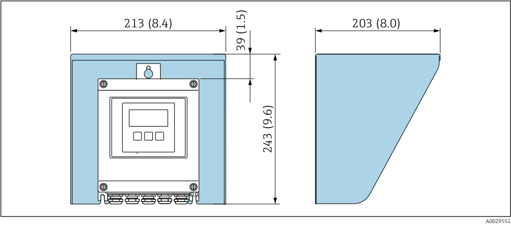
20 Защитный козырек от погодных явлений для Proline 500 – цифровое исполнение; мм (дюймах)
