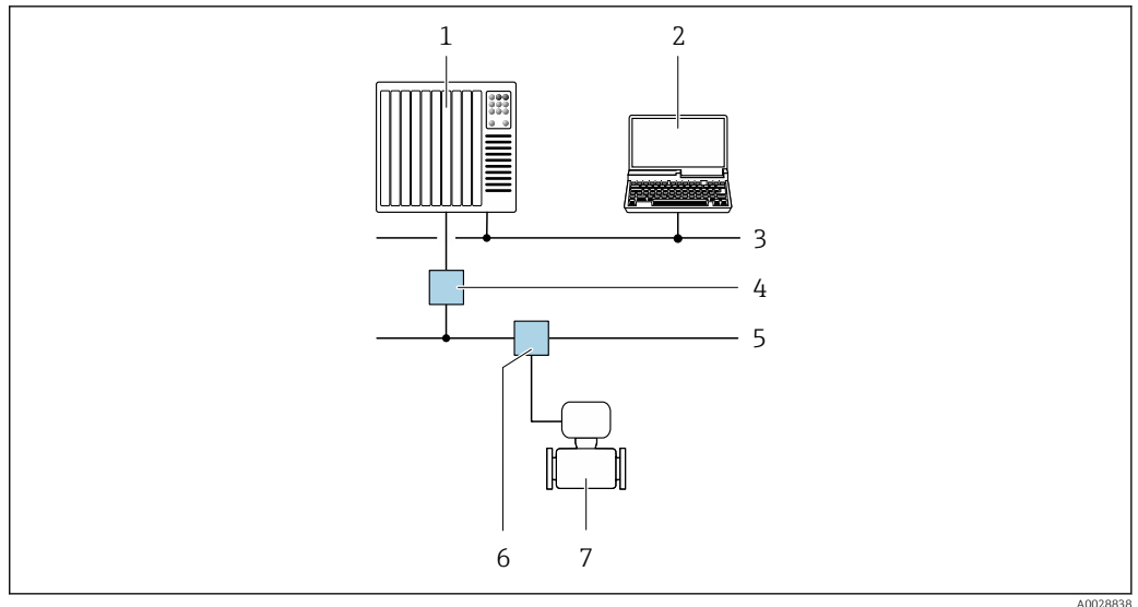
52 Варианты дистанционного управления по сети PROFIBUS PA
