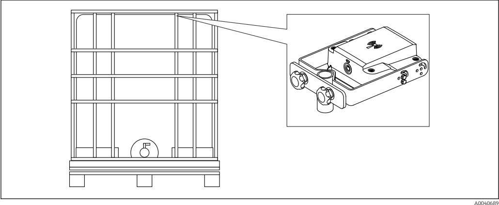
3 Montage mit Montagebügel Rohr/IBC
