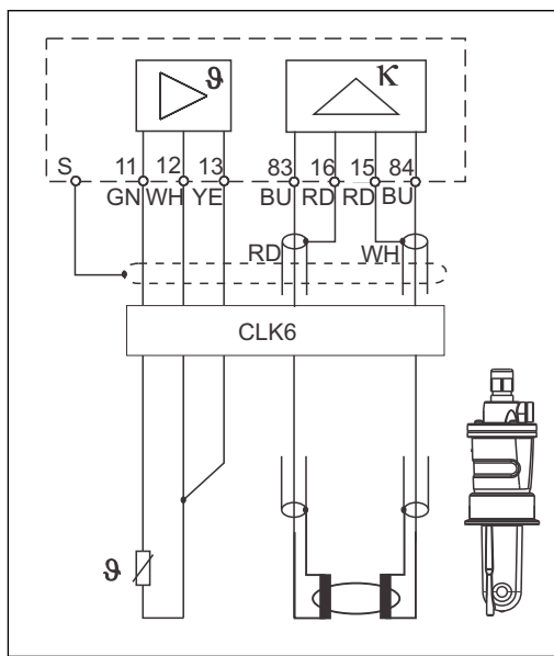
7 Tilkobling av induktive sensorer
