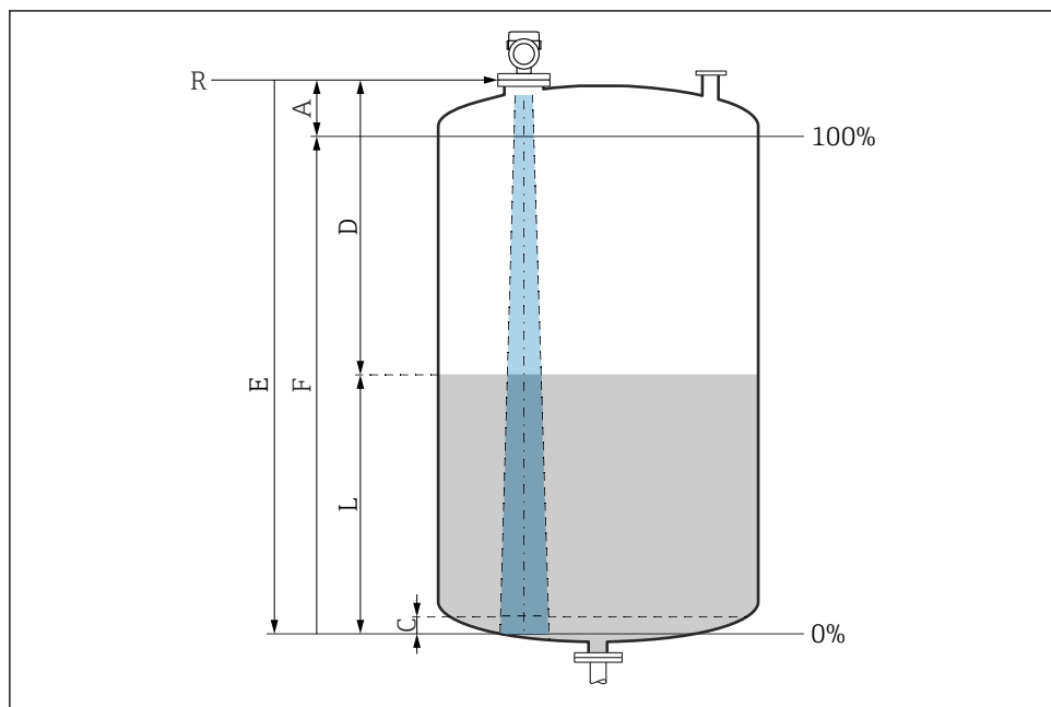
11 Parametri de configurare pentru măsurarea nivelului în lichide
