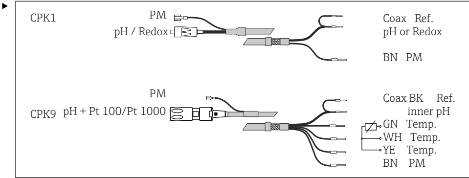
图 11 连接带 CPK1 或 CPK9 电缆的 pH/ORP 电极
