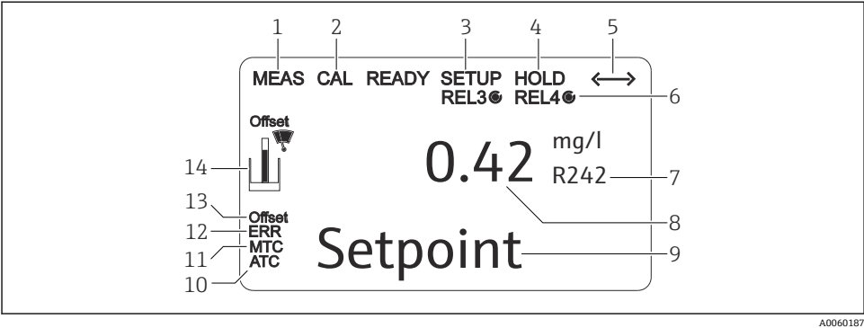
图 15 变送器的液晶显示屏
