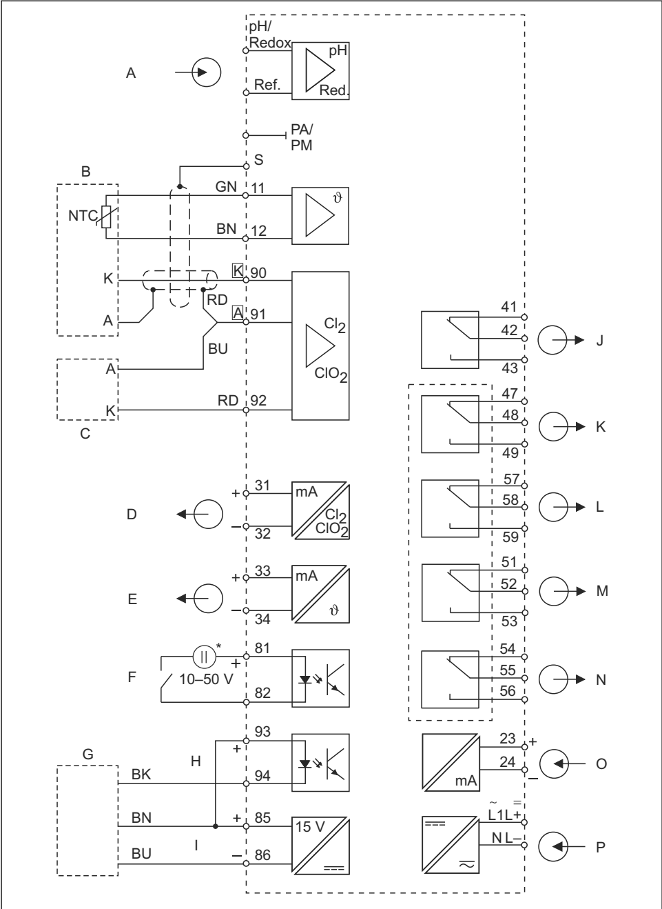
7 变送器 (类型 1) 的电气连接示意图
