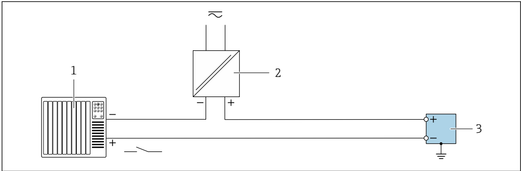
18 状态输入 1 自动化系统，带无源开关量输出（例如 PLC） 2 电源 3 变送器，带状态输入
