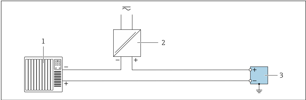
17 接线实例：继电器输出 1 自动化系统，带开关量输入（例如 PLC） 2 电源 3 变送器，带继电器输出
