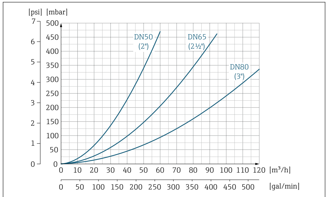
34 Configuraciones de pérdida de carga que incorporan adaptadores con diámetros nominales de DN 50 a 80 (2 a 3") para códigos de producto con opción para "Diseño", opción C "Brida fija, sin tramos rectos de entrada/salida"
