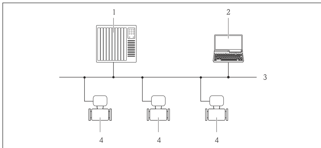
Fig. 23 Opciones para la configuración a distancia mediante red PROFIBUS DP
