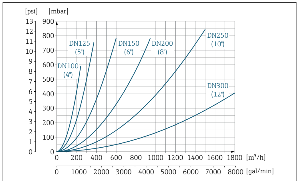
35 Configuraciones de pérdida de carga que incorporan adaptadores con diámetros nominales de DN 100 a 300 (4 a 12") para códigos de producto con opción para "Diseño", opción C "Brida fija, sin tramos rectos de entrada/salida"
