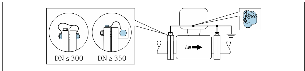
9 Igualación de potencial mediante borna de tierra y bridas de tubería
