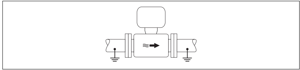
8 Igualación de potencial a través del tubo de medición
