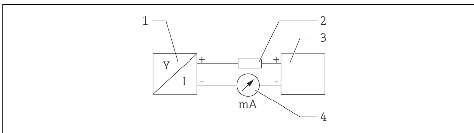
1 Schéma de principe du raccordement HART
