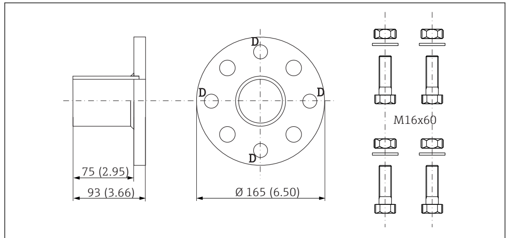
12 Connessione a saldare, dimensioni in mm (in)
