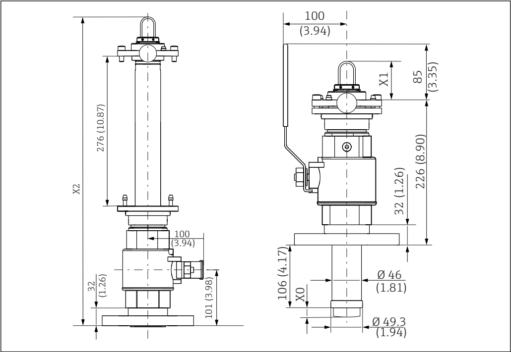
9 Dimensioni in mm (in)
