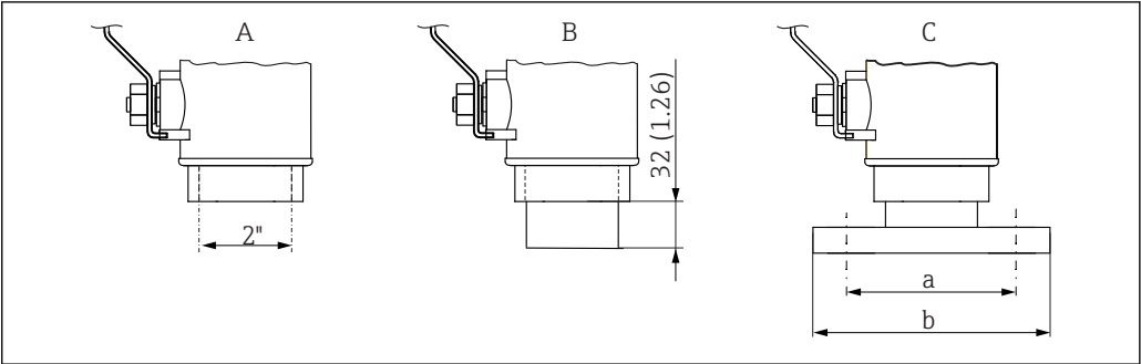
11 Dimensioni delle connessioni al processo in mm (in)
