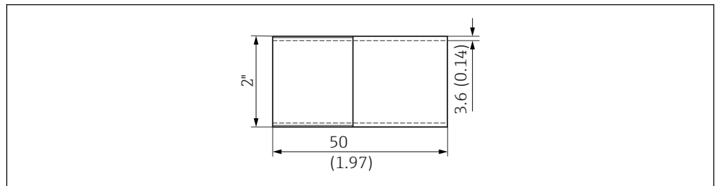
13 Niplo a saldare, dimensioni in mm (in)
