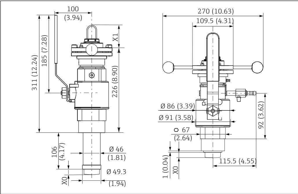
7 Dimensioni in mm (in) X0, Le dimensioni dipendono dal sensore X1
