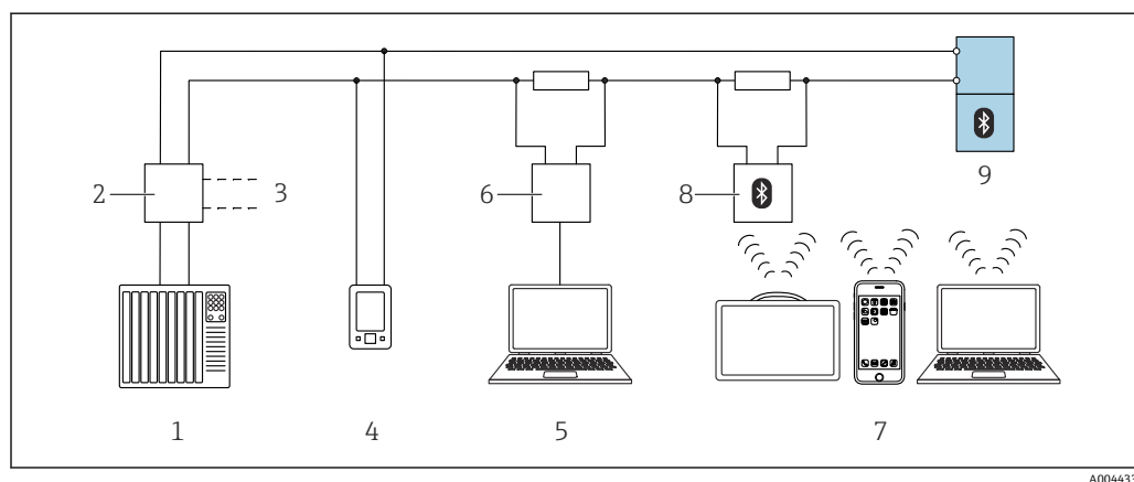
19 通过 HART 通信实现远程操作
