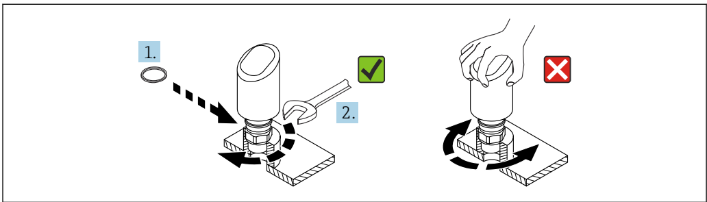
13 拧入设备
