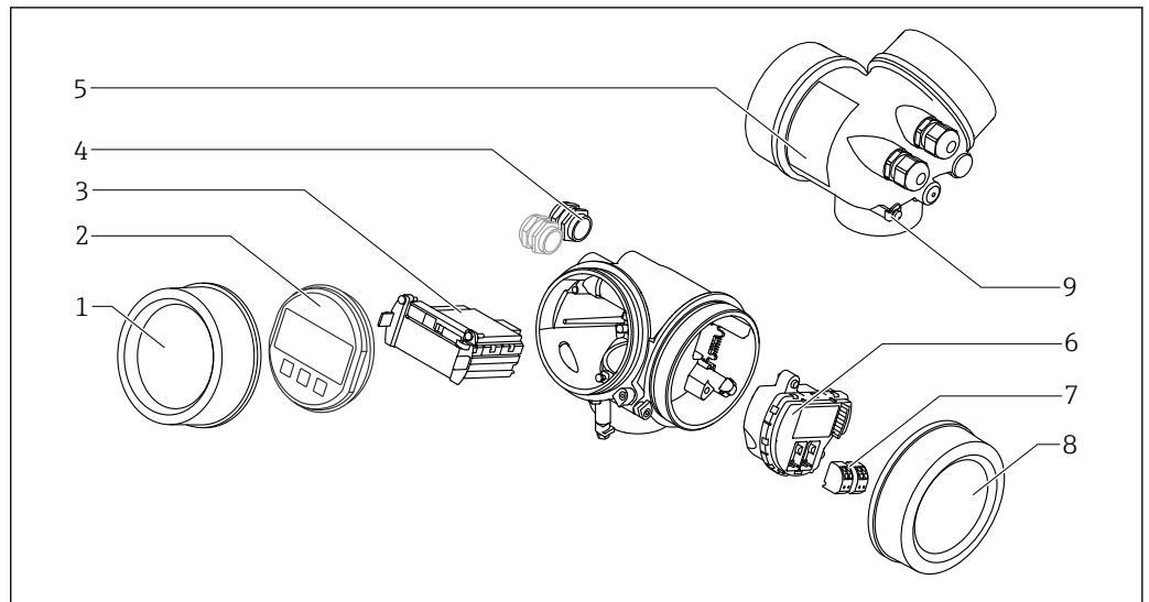
2 Aufbau des Elektronikgehäuses
