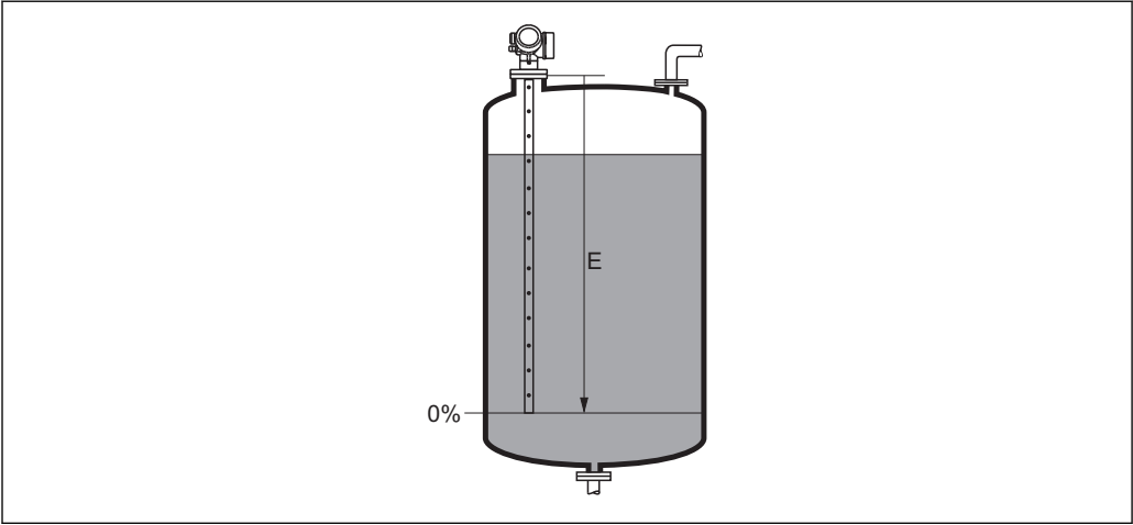
31 Abgleich Leer (E) bei Messungen in Flüssigkeiten
