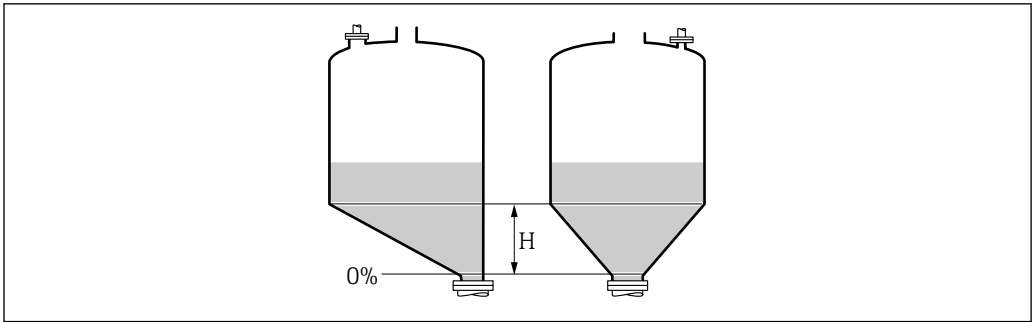
H Zwischenhöhe
