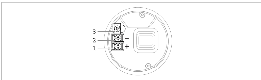
図 1 端子部の接続端子と接地端子
