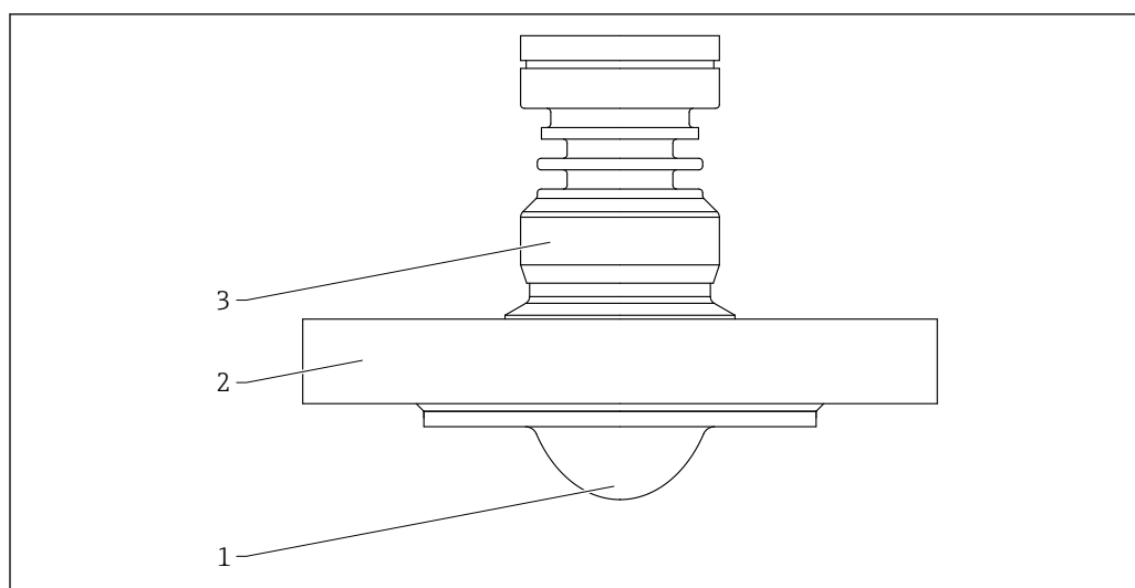
64 Materiale; rivestita, flush mounted, in PTFE, 50 mm (2 in), con flangia
