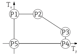
15 Custodia in plastica; temperatura di processo 0 ... +150 °C (+32 ... +302 °F) con approvazione CSA C/US
