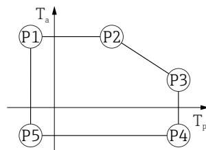
31 Custodia in alluminio; rivestita; temperatura di processo -20 ... +200 °C (-4 ... +392 °F)
