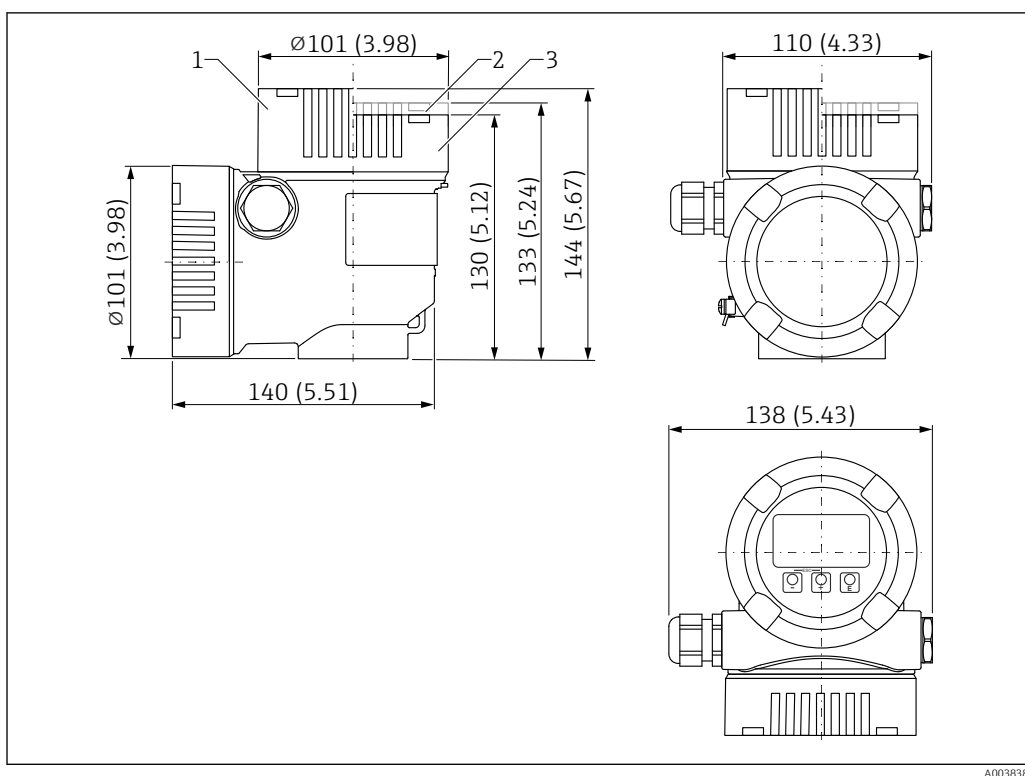
56 Dimensioni; custodia a vano doppio, a L, in alluminio, rivestita; completa di raccordo M20 e tappo in plastica. Unità di misura mm (in)
