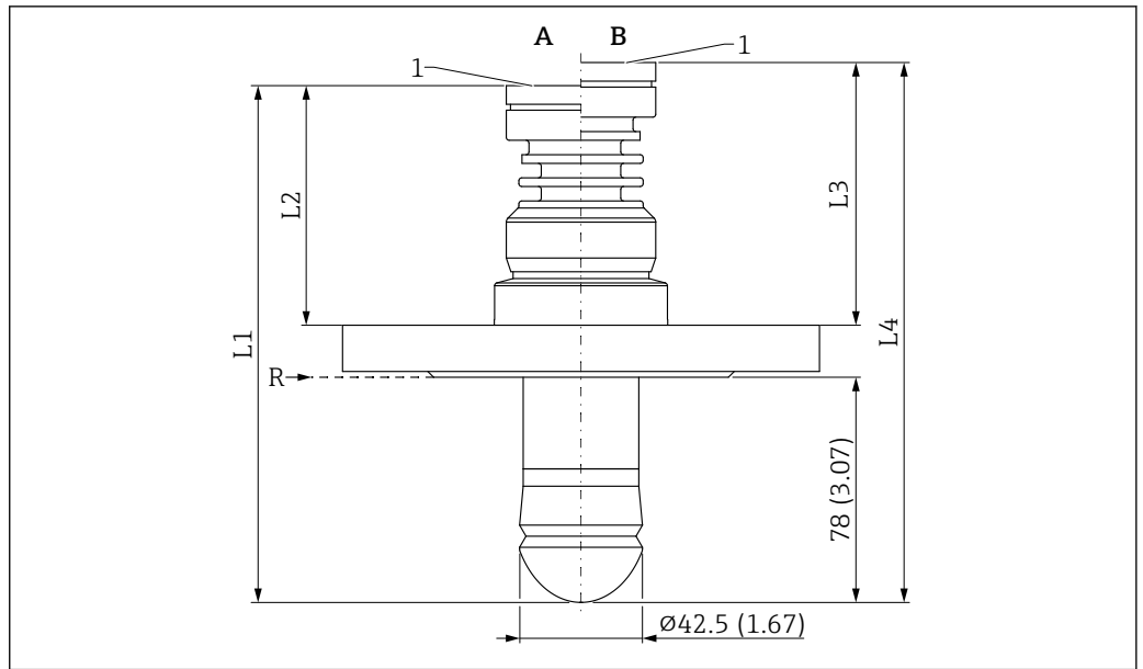
59 Dimensioni della flangia di connessione al processo. Unità di misura mm (in)
