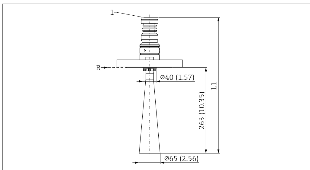
58 Dimensioni dell'antenna a cono DN65 - flangia di connessione al processo. Unità di misura mm (in)
