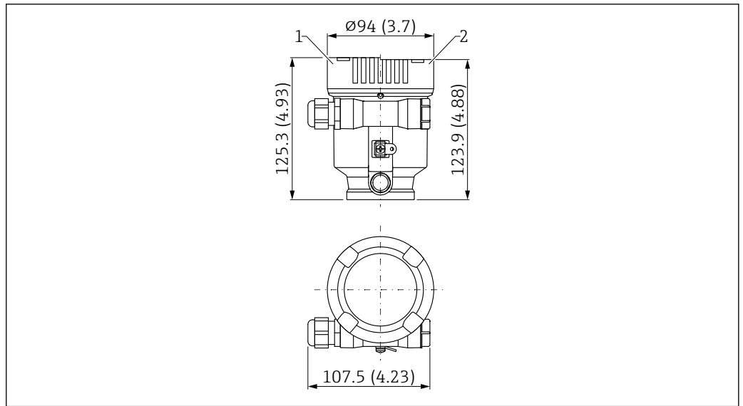
52 Dimensioni; custodia a vano unico, in plastica; completa di raccordo M20 e tappo in plastica. Unità di misura mm (in)
