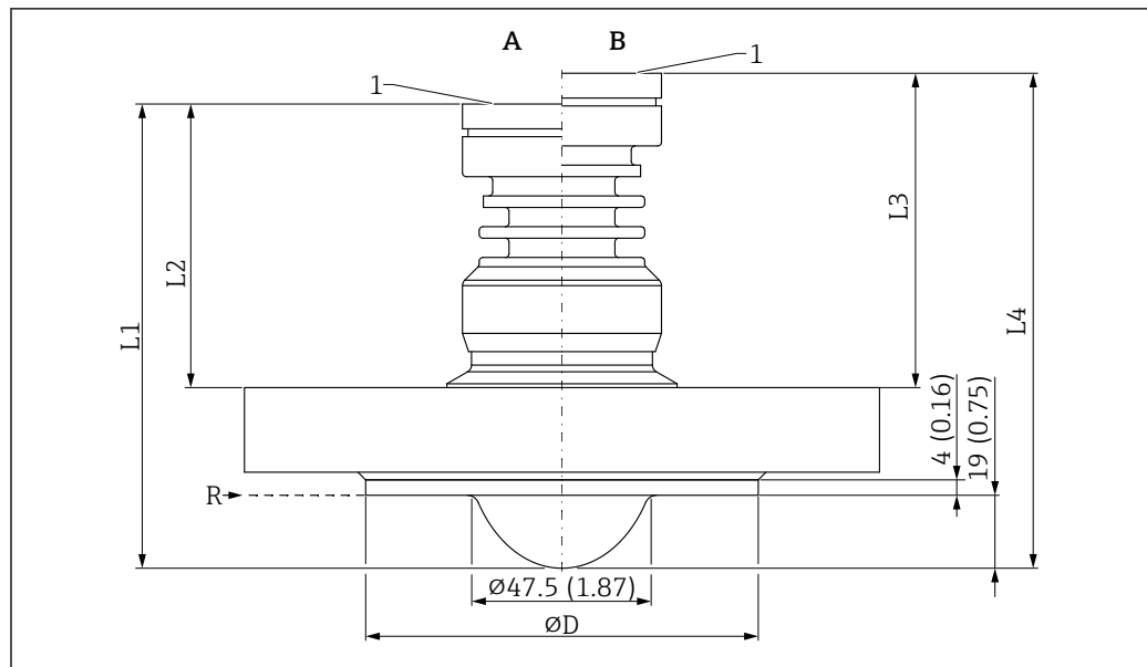
60 Dimensioni dell'antenna, flush-mounted con rivestimento, PTFE, 50 mm (2 in), con flangia. Unità di misura mm (in)
