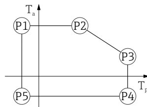
22 Custodia in plastica; temperatura di processo -40 \dots +280 \text{ }^{\circ}\text{C} ( -40 \dots +536 \text{ }^{\circ}\text{F} )
