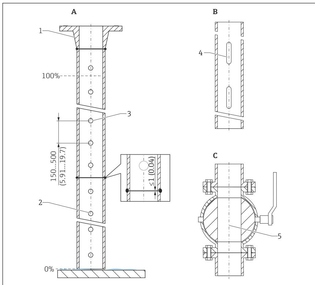
11 Esempio di design di un tubo di calma. Unità di misura mm (in)
