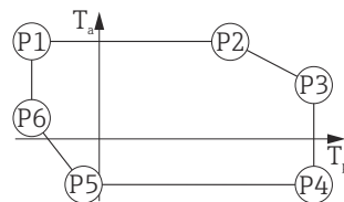
28 Custodia in plastica; temperatura di processo -196 \dots +200 \text{ }^{\circ}\text{C} ( -320 \dots +392 \text{ }^{\circ}\text{F} )
