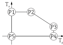
29 Approvazione CSA C/US e custodia in plastica; temperatura di processo 0 ... +200 °C (+32 ... +392 °F)
