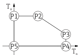
23 Custodia in plastica; temperatura di processo 0 ... +280 °C (+32 ... +536 °F) con approvazione CSA C/US
