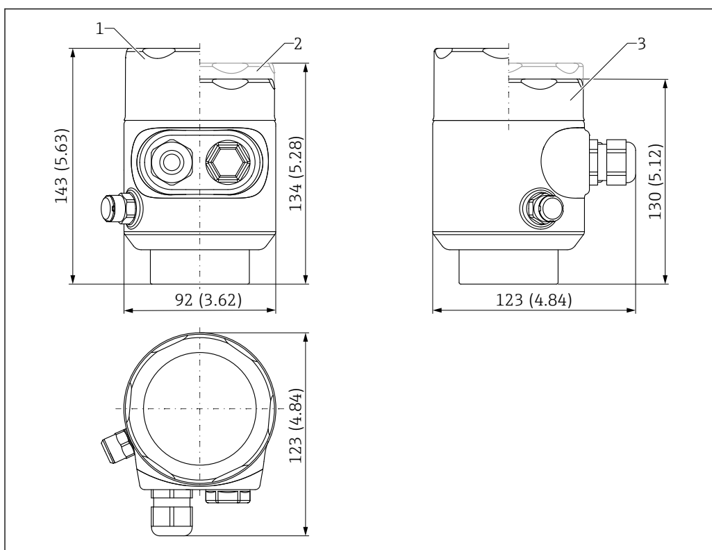
■ 54 Dimensioni; custodia a vano unico, 316L, igienica; completa di raccordo M20 e tappo in plastica. Unità di misura mm (in)
