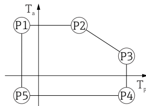
30 Custodia in alluminio; rivestita; temperatura di processo -20 ... +150 °C (-4 ... +302 °F)
