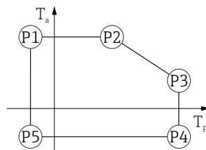
16 Custodia in plastica; temperatura di processo -20 ... +200 °C (-4 ... +392 °F)
