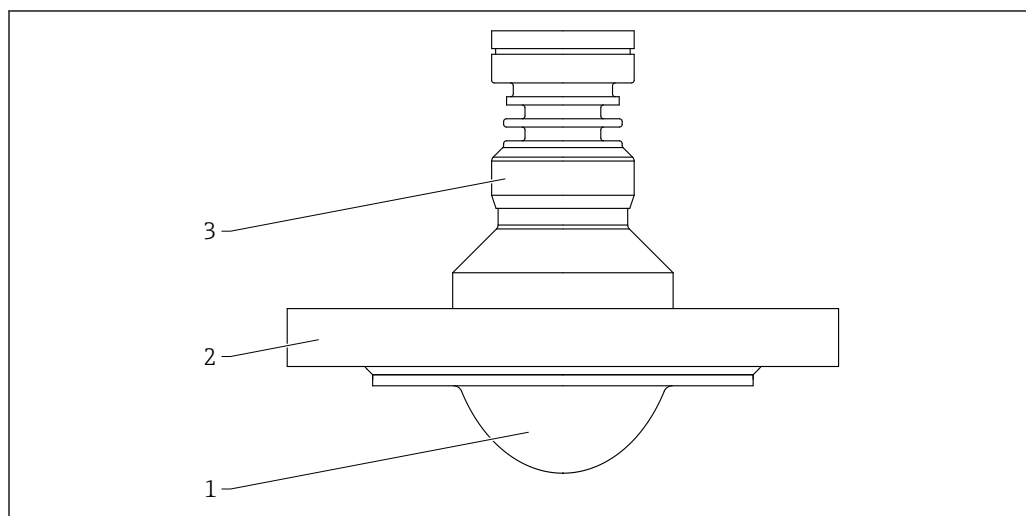
65 Materiale; rivestita, flush mounted, in PTFE, 80 mm (3 in), con flangia
