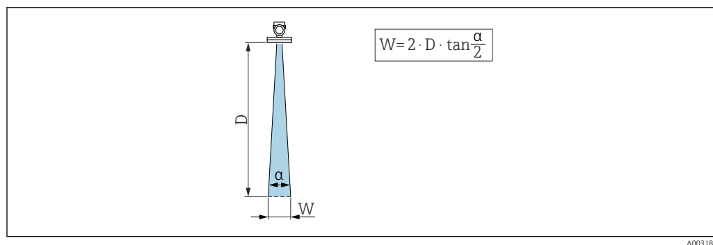
9 Rapporto tra angolo di emissione \alpha , distanza D e diametro del lobo di emissione W
