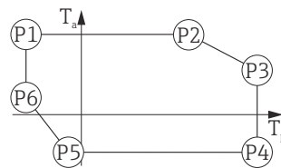
45 Custodia 316L; temperatura di processo -196 \dots +200 \text{ }^{\circ}\text{C} ( -320 \dots +392 \text{ }^{\circ}\text{F} )
