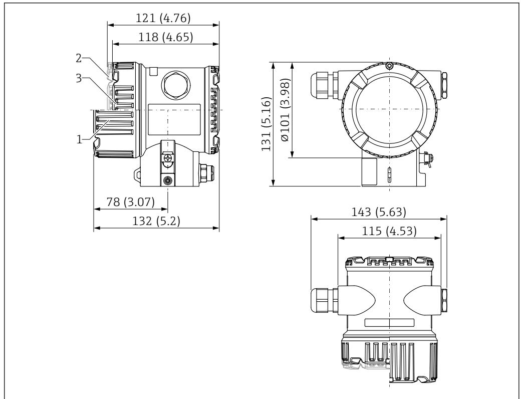
55 Dimensioni; custodia a vano doppio, in alluminio, rivestita; completa di raccordo M20 e tappo in plastica. Unità di misura mm (in)
