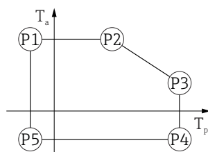
18 Custodia in plastica; temperatura di processo -40 ... +150 °C (-40 ... +302 °F)
