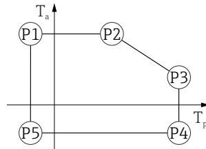
38 Custodia 316L; temperatura di processo -20 ... +150 °C (-4 ... +302 °F)
