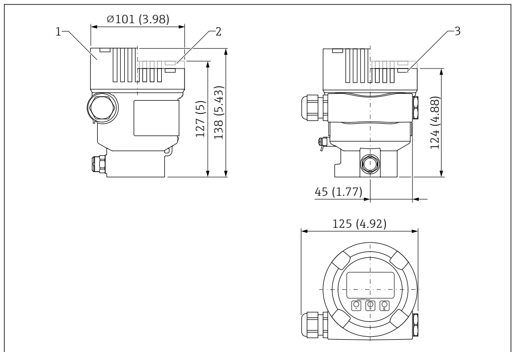
53 Dimensioni; custodia a vano unico, in alluminio, rivestita; completa di raccordo M20 e tappo in plastica. Unità di misura mm (in)
