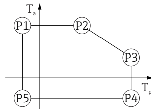
39 Custodia 316L; temperatura di processo -20 ... +200 °C (-4 ... +392 °F)
