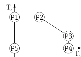
25 Custodia in plastica; temperatura di processo 0 ... +450 °C (+32 ... +842 °F) con approvazione CSA C/US
