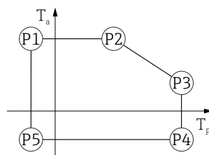
46 Custodia 316L; igienica; temperatura di processo -20 \dots +150 \text{ }^{\circ}\text{C} ( -4 \dots +302 \text{ }^{\circ}\text{F} )
