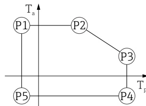
40 Custodia 316L; campo di temperature di processo: -40 ... +150 °C (-40 ... +302 °F)
