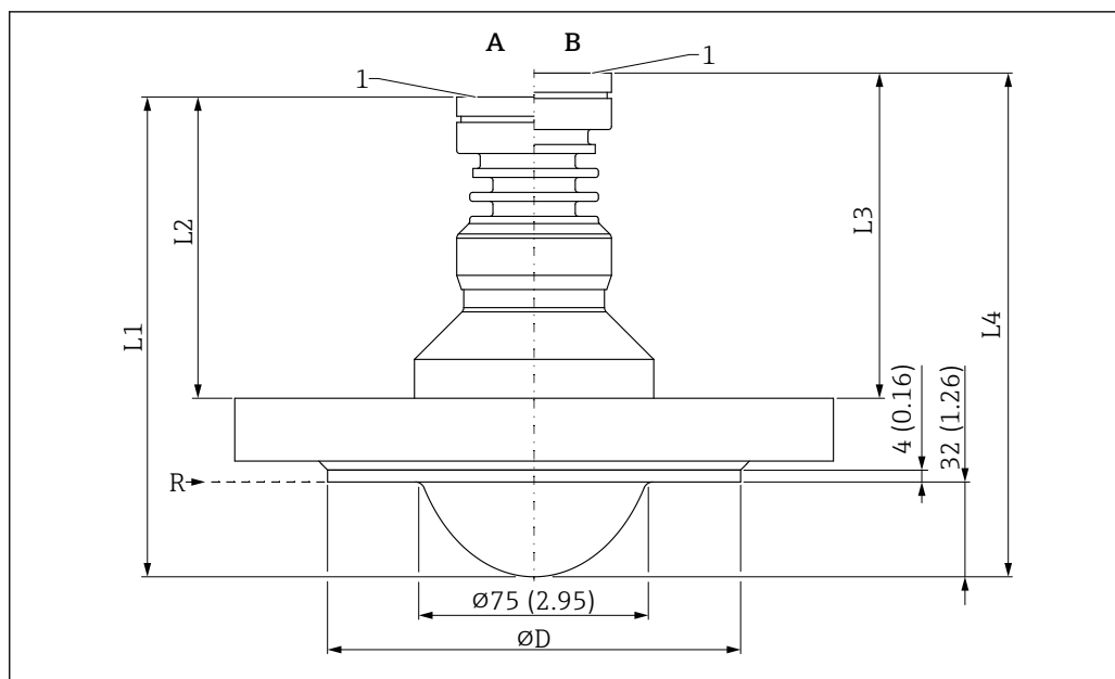
61 Dimensioni dell'antenna, flush-mounted con rivestimento, PTFE, 80 mm (3 in), con flangia. Unità di misura mm (in)
