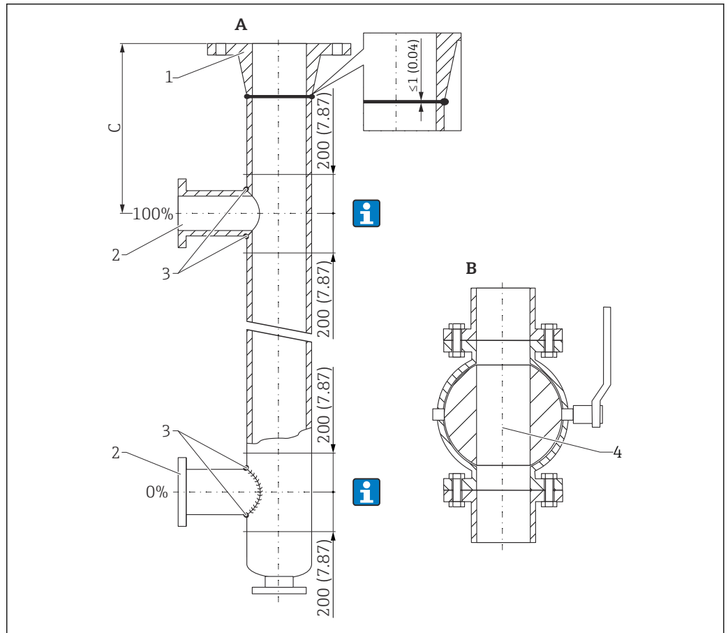
13 Esempio di design di un tubo bypass. Unità di misura mm (in)
