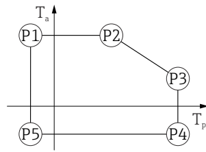
41 Custodia 316L; temperatura di processo -40 \dots +200 \text{ }^{\circ}\text{C} ( -40 \dots +392 \text{ }^{\circ}\text{F} )
